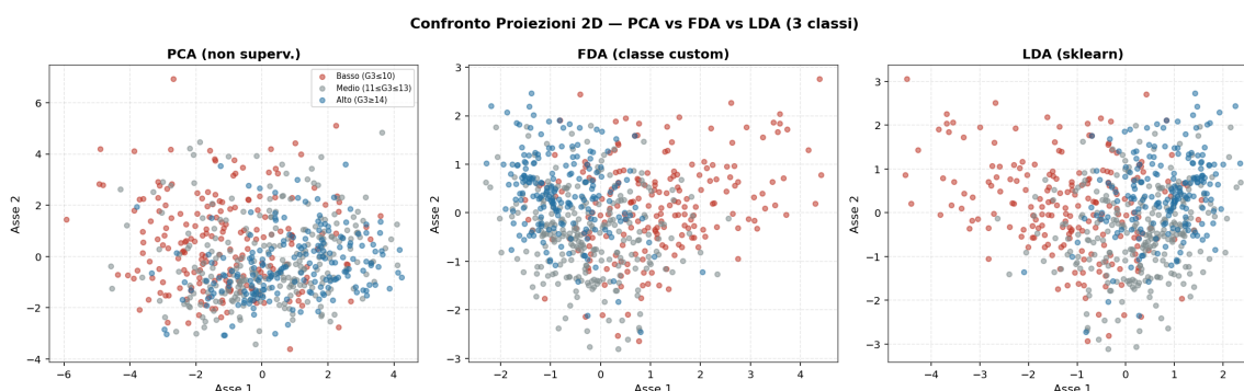
Figura 16: Confronto proiezioni 2D: PCA vs FDA vs LDA (3 classi).
