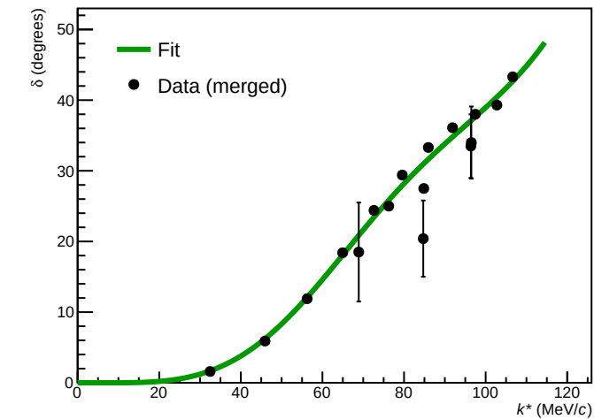
L=1, S=0 ( ^3P_0 )
