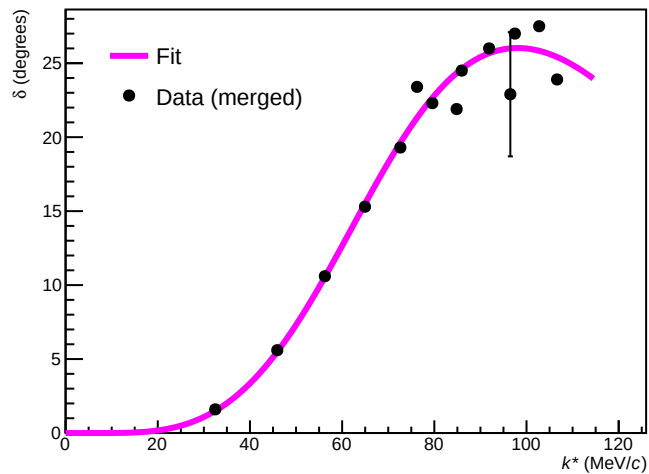
L=1, S=1 ( ^3P_1 )
