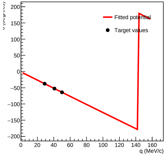
s=3/2 (quartet)
