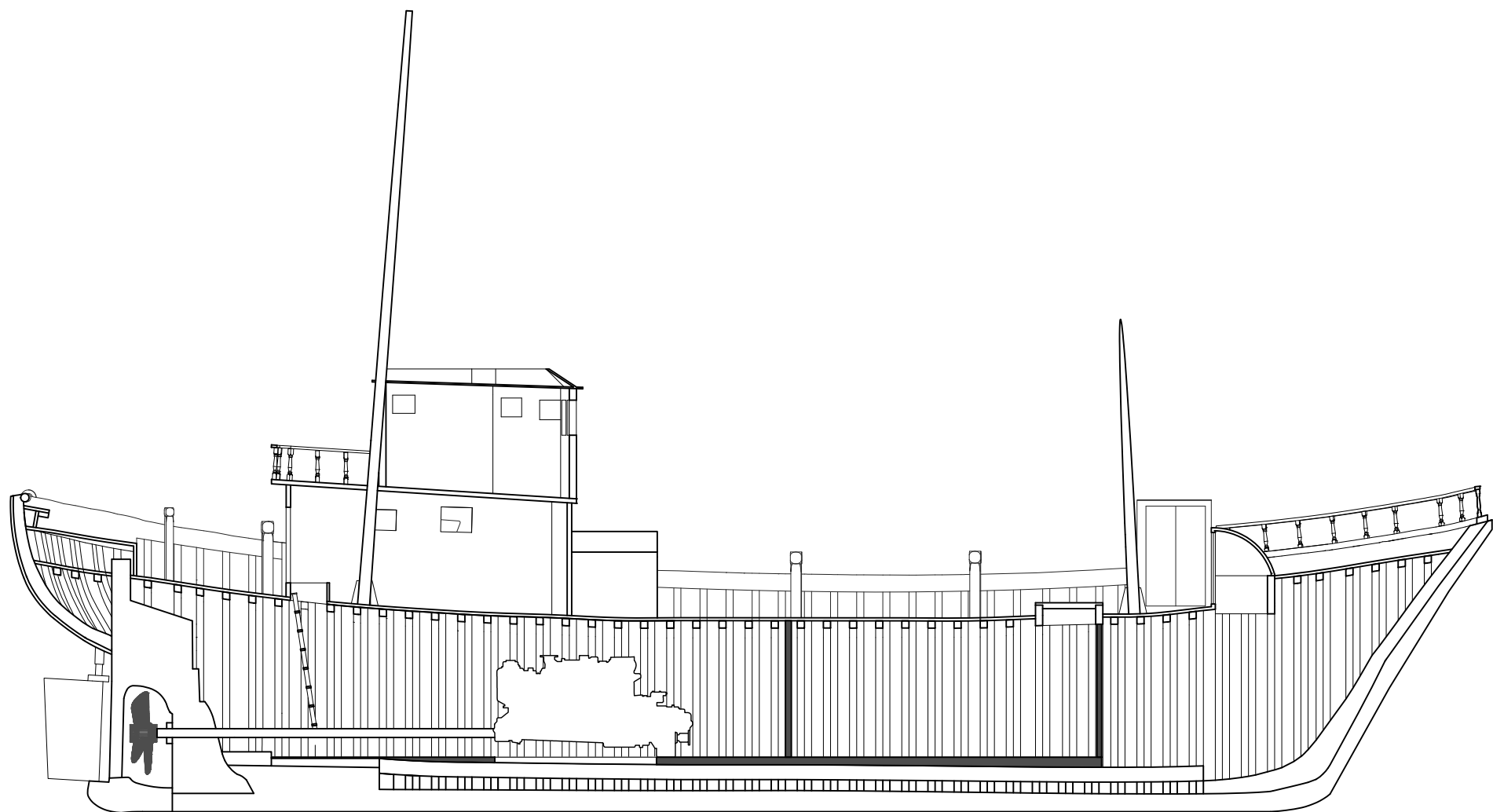
Longitudinal Section
