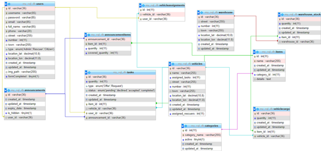
Σχήμα 1: Σχεσιακό Διάγραμμα ΒΔ
