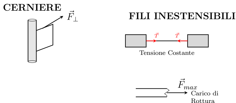
Figura 2.9: Esempi di forze vincolari: cerniere che esercitano forze perpendicolari all'asse e fili che trasmettono tensioni.
