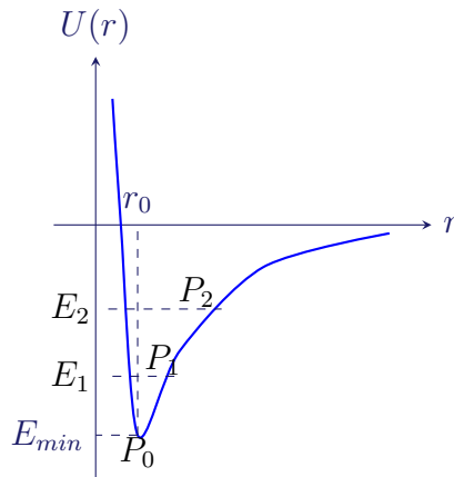
Figura 8.4: Curva dell'energia potenziale molecolare
