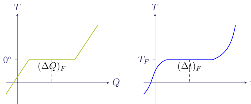
Figura 8.5: Grafici Temperatura-Calore e Temperatura-tempo per un cambiamento di stato
