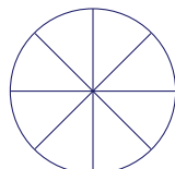
Corpo Nero
