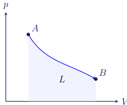
Figura 8.7: Lavoro termodinamico come area sottesa nel piano di Clapeyron ( p - V ).
