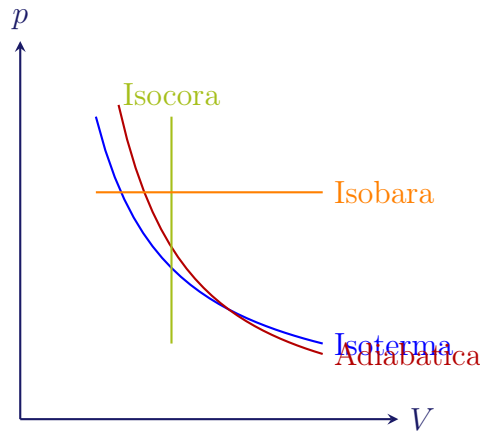
Figura 8.9: Confronto tra trasformazioni nel piano p - V .
