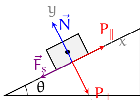
Figura 20: Equilibrio limite su piano inclinato.
