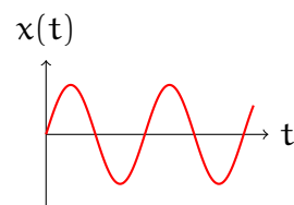
Funzione Armonica
