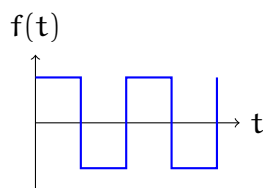
Funzione Periodica
