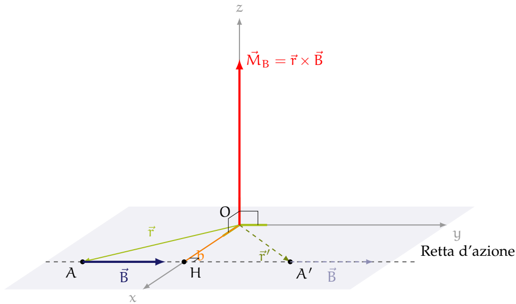
Figura 30: Rappresentazione vettoriale del momento di un vettore \vec{B} rispetto al polo O. Sulla retta d'azione sono evidenziati i punti arbitrari A e A' ed il braccio b.
