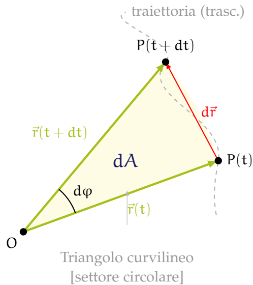
Figura 33: Significato geometrico della velocità areolare: il raggio vettore spazza l'area infinitesima dA nell'intervallo dt .
