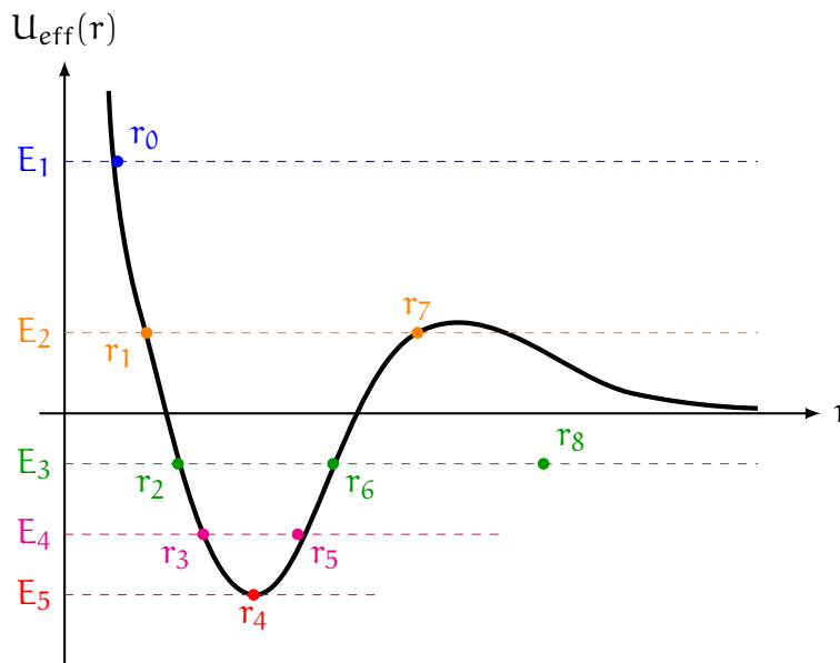
Figura 34: Grafico qualitativo del Potenziale Efficace con vari livelli di Energia E_0 , che mostra le radici (punti di inversione r_i ) e delimita le regioni accessibili al moto.
