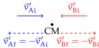
Figura 29: Inversione delle velocità nel sistema del CM per un urto elastico unidimensionale.
