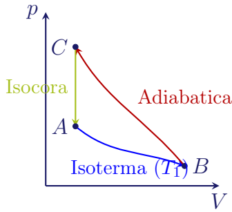
Figura 8.13: Ciclo monoterme costituito da un'isoterma reversibile, un'adiabatica reversibile e un'isocora irreversibile.
