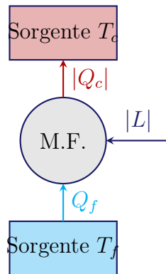
Figura 8.12: Schema di principio di una macchina frigorifera.
