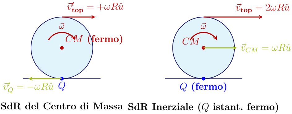
Figura 7.7: Confronto tra le descrizioni cinematiche del puro rotolamento: nel sistema del Centro di Massa il disco compie una pura rotazione ed il punto Q arretra con velocità -\omega R ; nel sistema inerziale il punto Q è istantaneamente fermo e il Centro di Massa trasla con velocità \omega R .
