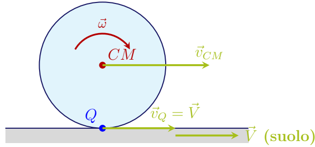
Figura 7.8: Puro rotolamento su una superficie mobile: affinché non vi sia slittamento, la velocità istantanea del punto di contatto Q deve eguagliare la velocità di traslazione \vec{V} della superficie d'appoggio.
