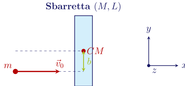
Figura 7.18: Geometria dell'urto tra un proiettile di massa m con velocità \vec{v}_0 e una sbarretta libera di massa M e lunghezza L , con parametro d'impatto b rispetto al centro di massa.
