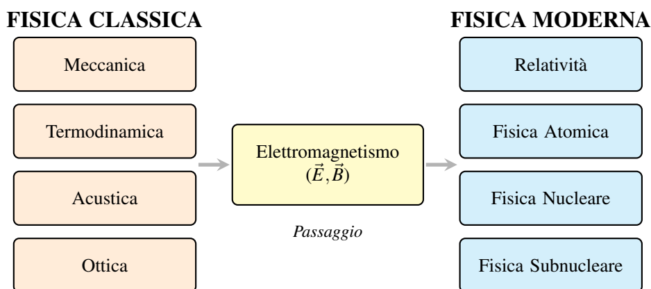
Figura 1.2: Lo sviluppo storico dalla Fisica Classica alla Moderna.
