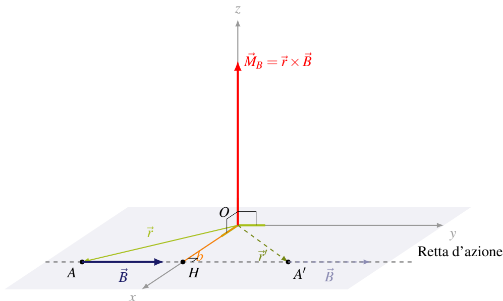
Figura 5.1: Rappresentazione vettoriale del momento di un vettore \vec{B} rispetto al polo O . Sulla retta d'azione sono evidenziati i punti arbitrari A e A' ed il braccio b .
