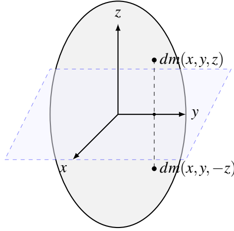
Figura 7.3: Rappresentazione di un corpo tagliato dal suo piano di simmetria equatoriale.
