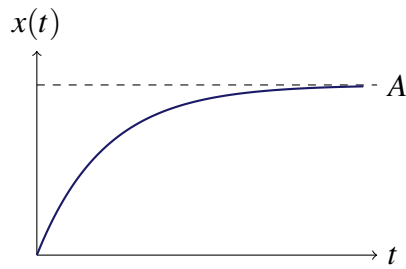
Figura 1.6: Andamento della posizione nel moto smorzato: tende asintoticamente ad A.
