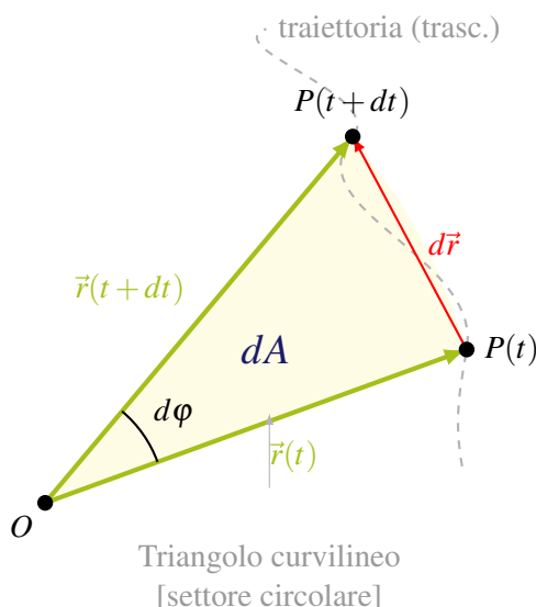
Figura 5.4: Significato geometrico della velocità areolare: il raggio vettore spazza l'area infinitesima dA nell'intervallo dt .
