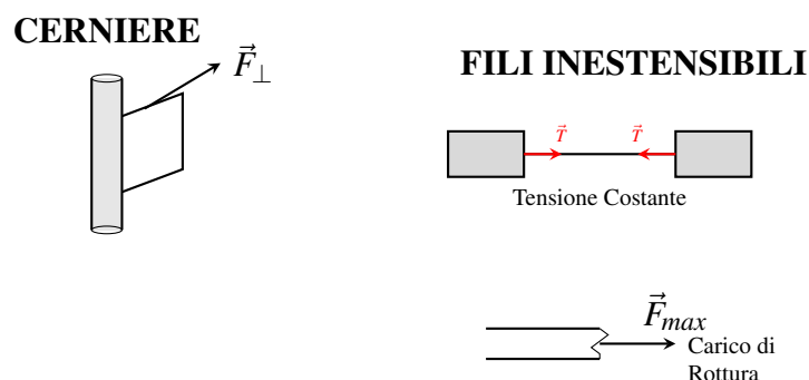
Figura 2.9: Esempi di forze vincolari: cerniere che esercitano forze perpendicolari all'asse e fili che trasmettono tensioni.
