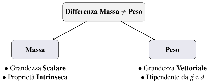
Figura 2.6: Schema delle differenze fondamentali tra Massa e Peso.
