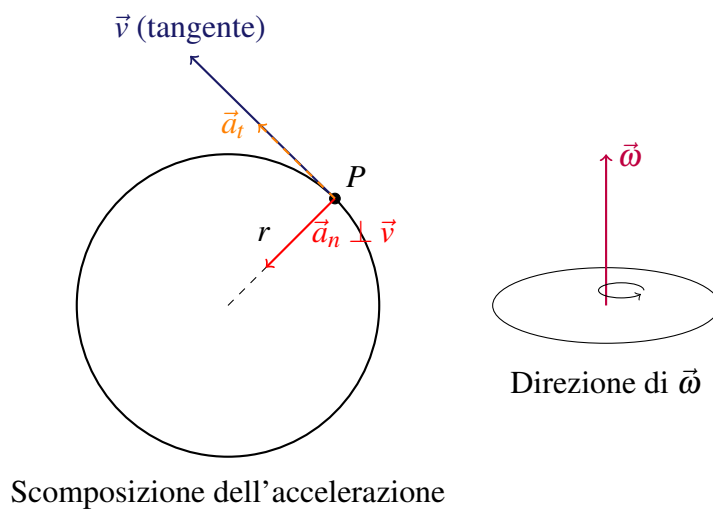
Figura 1.7: Cinematica del moto circolare.
