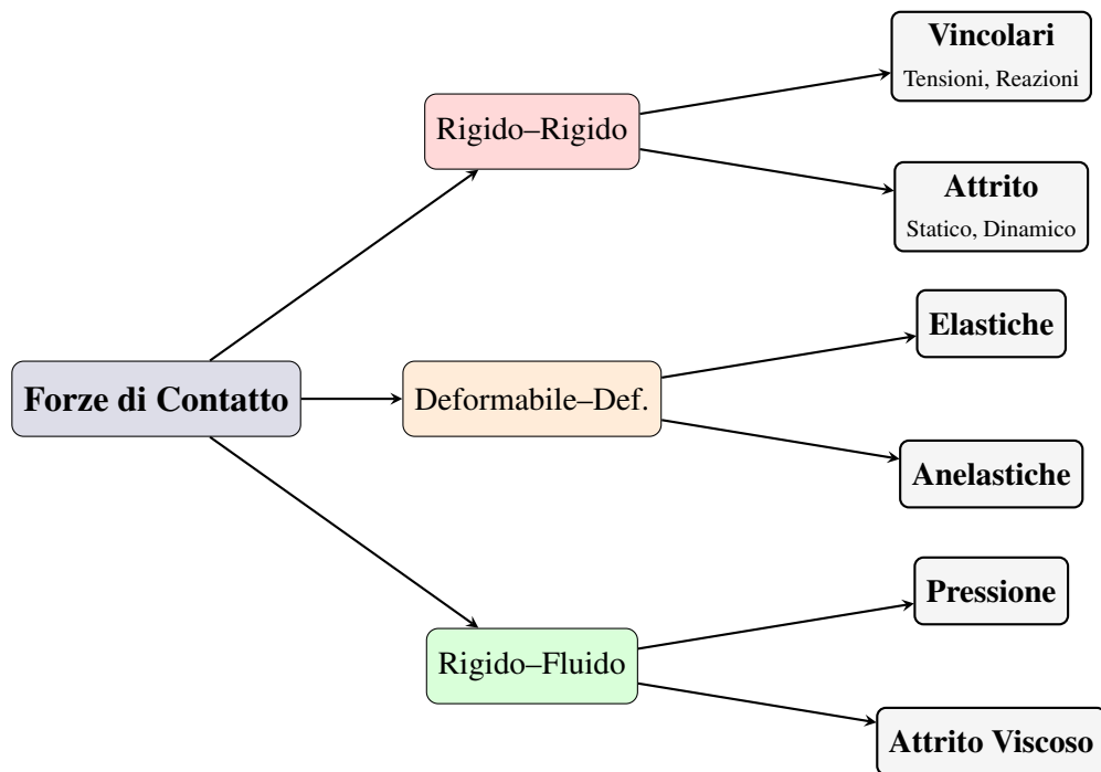
Figura 2.1: Classificazione delle Forze di Contatto.
