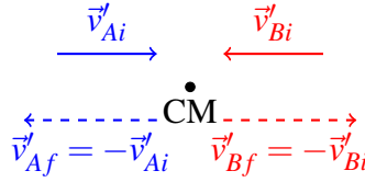
Figura 4.4: Inversione delle velocità nel sistema del CM per un urto elastico unidimensionale.
