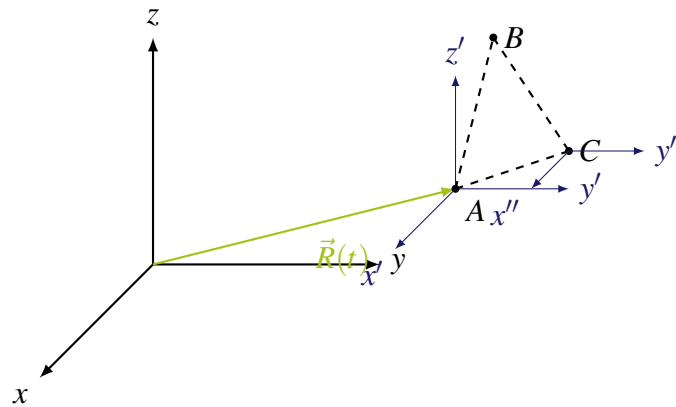
Figura 7.1: Costruzione incrementale dei gradi di libertà per tre punti non allineati del corpo rigido.
