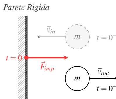
Figura 2.3: Urto elastico contro una parete rigida. La forza impulsiva \vec{F}_{imp} agisce per \Delta t \rightarrow 0 , causando la variazione di quantità di moto \Delta\vec{p} = \vec{p}(0^+) - \vec{p}(0^-) .
