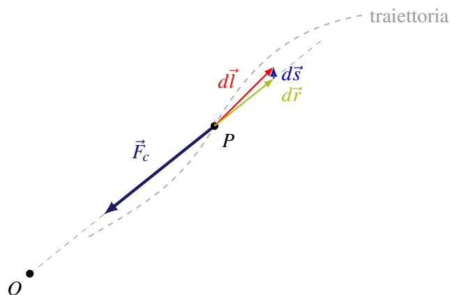
Figura 5.3: Scomposizione dello spostamento elementare d\vec{l} in componente radiale ( d\vec{r} ) e trasversale ( d\vec{s} ) per una forza centrale \vec{F}_c .
