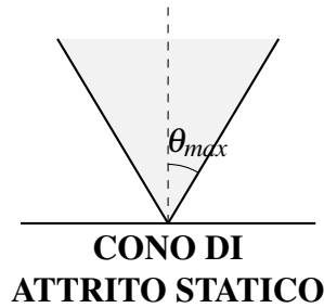
Figura 2.14: Cono di Attrito.
