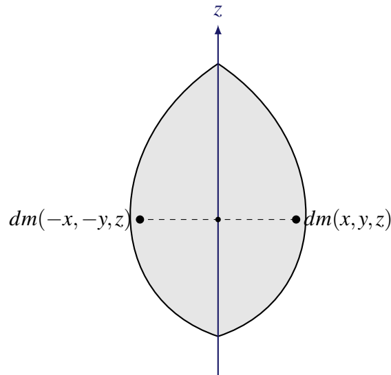
Figura 7.2: Corpo con asse di simmetria z . Ad ogni elemento di massa ad una certa distanza dall'asse corrisponde un elemento identico dalla parte opposta.
