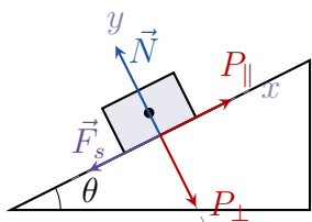
Figura 2.13: Equilibrio limite su piano inclinato.
