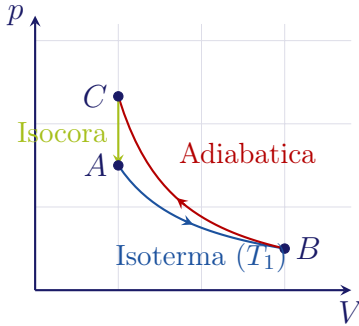
Figura 8.30: Ciclo monoterma costituito da un'isoterma reversibile ( A \rightarrow B ), un'adiabatica reversibile ( B \rightarrow C ) e un'isocora irreversibile ( C \rightarrow A ).
