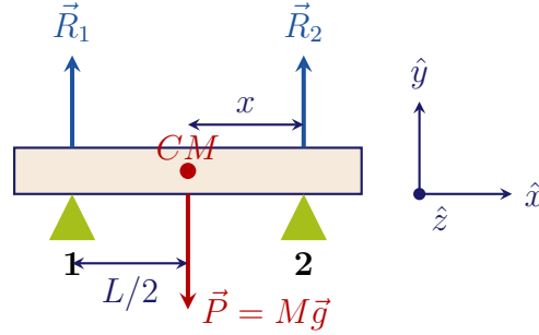
Figura 7.25: Equilibrio di una trave soggetta alla forza peso \vec{P} e a due reazioni vincolari \vec{R}_1 e \vec{R}_2 . L'equilibrio rotazionale impone limiti precisi alla posizione x del secondo appoggio affinché le reazioni vincolari risultino concordi al verso di appoggio.
