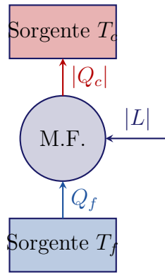
Figura 8.27: Schema di principio di una macchina frigorifera.
