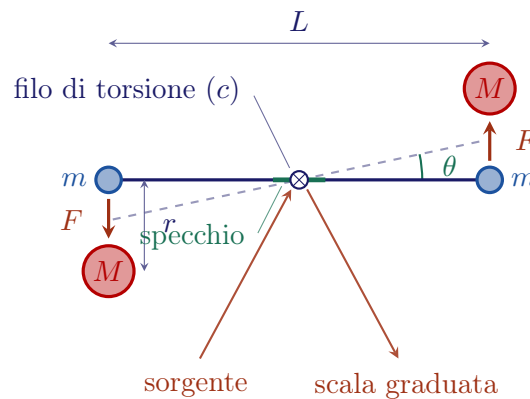
Figura 6.2: Schema della bilancia di torsione di Cavendish, vista dall'alto. Le due grandi masse M sono disposte da lati opposti dell'asticella, così che le attrazioni sulle masse m formino una coppia : essa torce il filo di un angolo \theta , finché la reazione elastica non la equilibra. Un raggio luminoso riflesso da uno specchio solidale con l'asticella amplifica la rotazione fino a renderla leggibile su una scala graduata distante.
