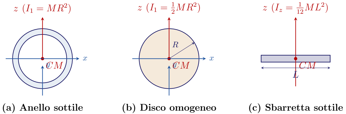
Figura 7.12: Momenti d'inerzia di corpi continui omogenei monodimensionali e bidimensionali rispetto all'asse principale d'inerzia z passante per il Centro di Massa e ortogonale alla geometria del corpo.
