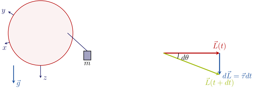
(a) Giroscopio simmetrico con massa esterna m applicata all'asse.
