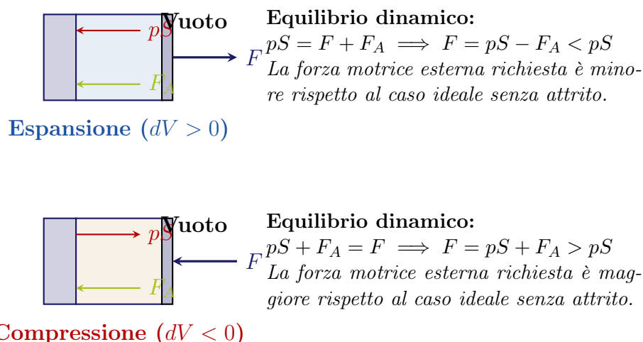
Figura 8.20: Confronto meccanico tra espansione e compressione di un gas in un cilindro con pistone in presenza di forza d'attrito viscoso F_A : l'isteresi meccanica dimostra l'irreversibilità dei processi reali.
