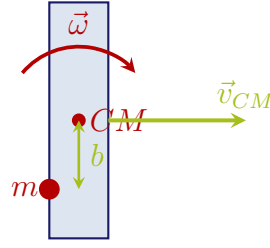
Figura 7.19: Stato finale nell'urto totalmente anelastico: il proiettile rimane conficcato nella sbarretta a distanza b dal centro di massa iniziale, formando un unico corpo rigido che ruototrasla con velocità \vec{v}_{CM} e velocità angolare \omega .
