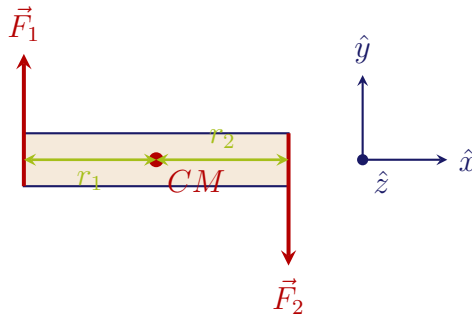
Figura 7.24: Coppia di forze: un sistema di forze a risultante nulla ( \vec{F}_1 = -\vec{F}_2 ) esercita un momento risultante non nullo \vec{\tau} = -LF\hat{z} , generando una rotazione pura attorno al centro di massa senza alcuna traslazione ( \vec{a}_{CM} = \vec{0} ).
