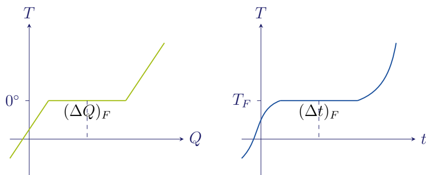
Figura 8.12: Grafici Temperatura-Calore e Temperatura-tempo per un cambiamento di stato
