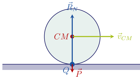
Figura 7.26: Equilibrio dinamico in puro rotolamento orizzontale: in assenza di forze trainanti esterne, la forza normale \vec{R}_N e la forza peso \vec{P} sono perfettamente allineate lungo la verticale passante per CM e Q . L'attrito statico è nullo ( f_s = 0 ) e il moto prosegue a velocità \vec{v}_{CM} costante senza dissipazione.
