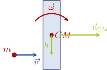
Figura 7.20: Stato finale nell'urto totalmente elastico: l'energia cinetica si conserva e il proiettile emerge con velocità residua \vec{v}' , mentre la sbarretta acquisisce velocità di traslazione \vec{v}_{CM} e velocità angolare \omega .
