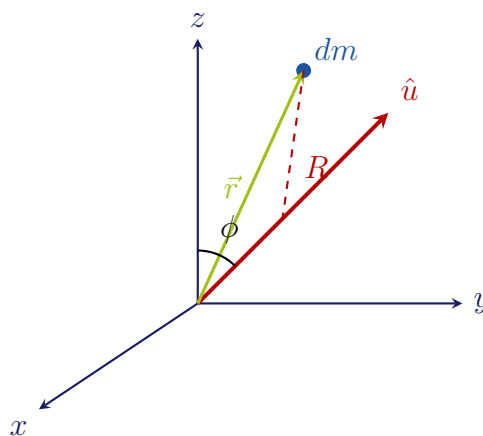
Figura 7.29: Calcolo del momento d'inerzia rispetto ad un asse \hat{u} : la distanza perpendicolare R dell'elemento di massa dm dall'asse di rotazione è data dal modulo del prodotto vettoriale \|\vec{r} \times \hat{u}\| = r \sin \phi .
