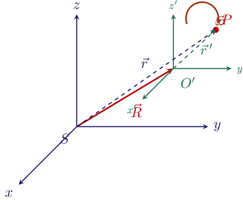
Figura 10.3: Composizione delle posizioni fra il sistema inerziale S e il sistema rototraslante S' , quest'ultimo animato dalla velocità angolare \vec{\omega} .
