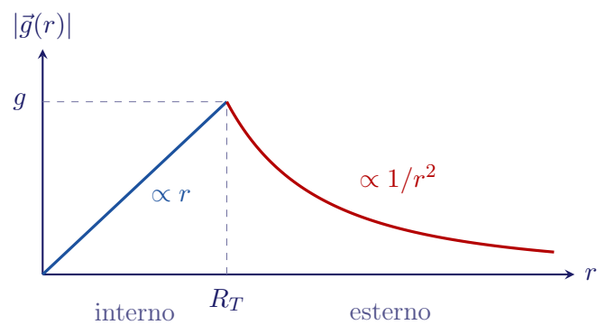
Figura 6.6: Modulo del campo gravitazionale generato da una sfera piena omogenea in funzione della distanza dal centro. Il campo cresce linearmente all'interno, raggiunge il massimo g sulla superficie e decresce come 1/r^2 all'esterno.
