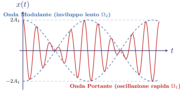
Figura 7.37: Rappresentazione del fenomeno dei battimenti: un'onda rapida la cui ampiezza varia lentamente nel tempo.
