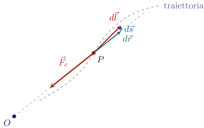
Figura 5.3: Scomposizione dello spostamento elementare d\vec{l} in componente radiale d\vec{r} e trasversale d\vec{s} . La forza centrale \vec{F}_c , parallela a \hat{r} , compie lavoro soltanto sulla prima.
