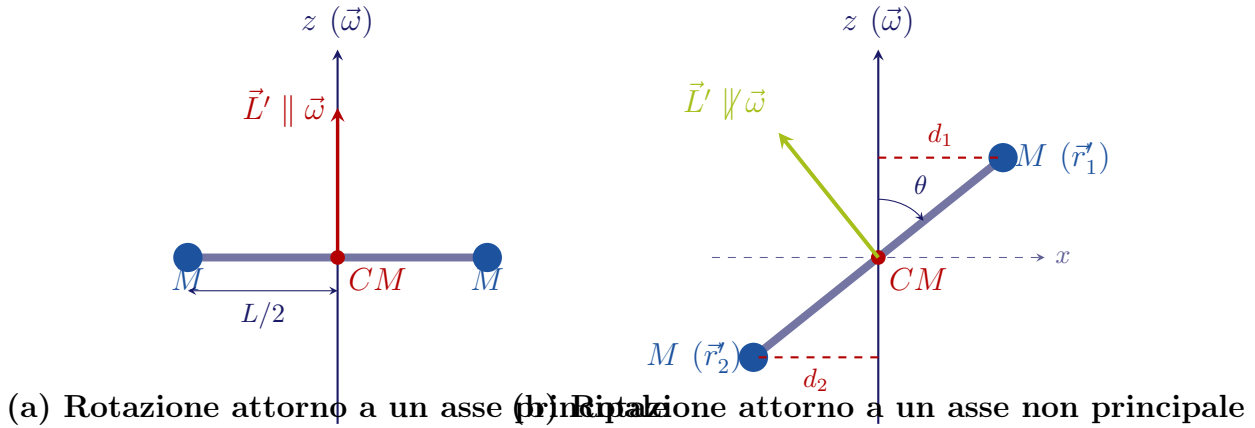
Figura 7.11: Esercizio del manubrio rotante: se l'asse di rotazione è ortogonale all'asta (caso a), esso è un asse principale d'inerzia e il momento angolare è parallelo a \vec{\omega} . Se l'asse è inclinato (caso b), compaiono componenti trasversali che rendono \vec{L}' non parallelo a \vec{\omega} , richiedendo una coppia di forze esterne sui vincoli per mantenere stabile l'asse.
