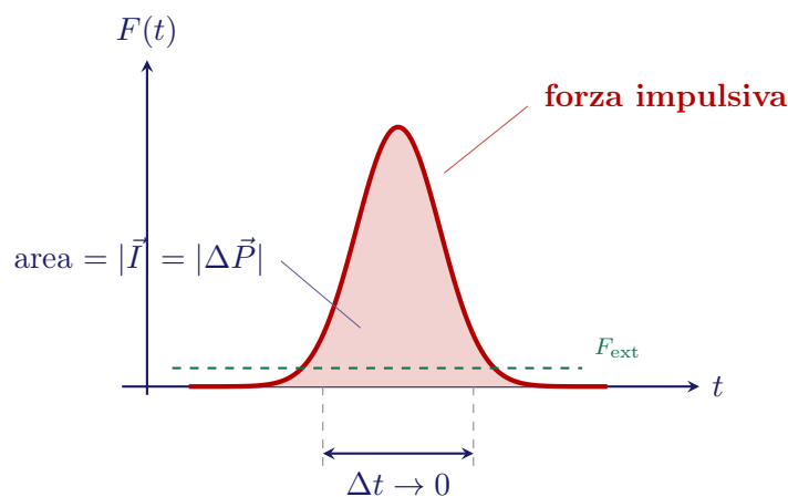
Figura 4.2: Andamento temporale di una forza impulsiva. L'area sottesa dalla curva è l'impulso \vec{I} = \Delta\vec{P} . In tratteggio verde, per confronto, una forza esterna ordinaria: il suo modulo è incomparabilmente più piccolo e, sull'intervallo \Delta t \rightarrow 0 , l'area che essa sottende è trascurabile.
