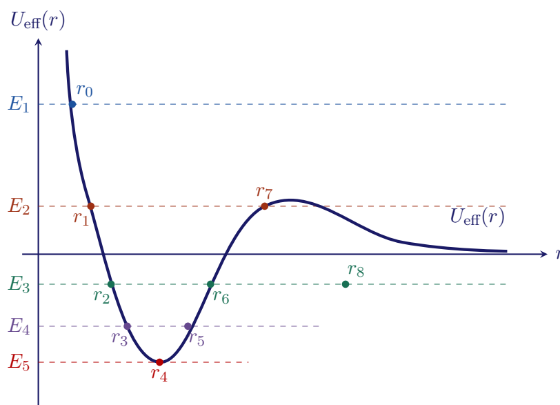
Figura 5.5: Andamento qualitativo del potenziale efficace e classificazione delle orbite. Ogni livello orizzontale rappresenta un valore dell'energia totale; le sue intersezioni con la curva sono i punti di inversione r_i , che delimitano le regioni accessibili al moto.
