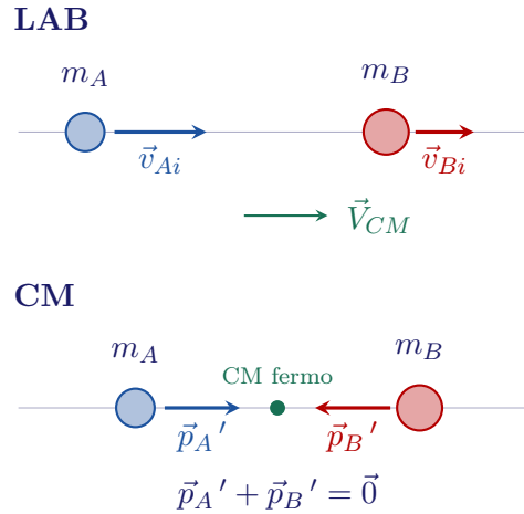
Figura 4.3: Lo stesso urto visto dal laboratorio e dal centro di massa. Nel LAB le due quantità di moto sono indipendenti; nel CM sono per costruzione uguali e opposte, e il centro di massa resta immobile prima, durante e dopo l'urto.
