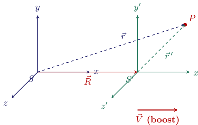
Figura 9.1: I due sistemi di riferimento adottati nello studio dei moti relativi: il sistema assoluto S e il sistema relativo S' , traslato di \vec{R} e animato dalla velocità di trascinamento \vec{V} .
