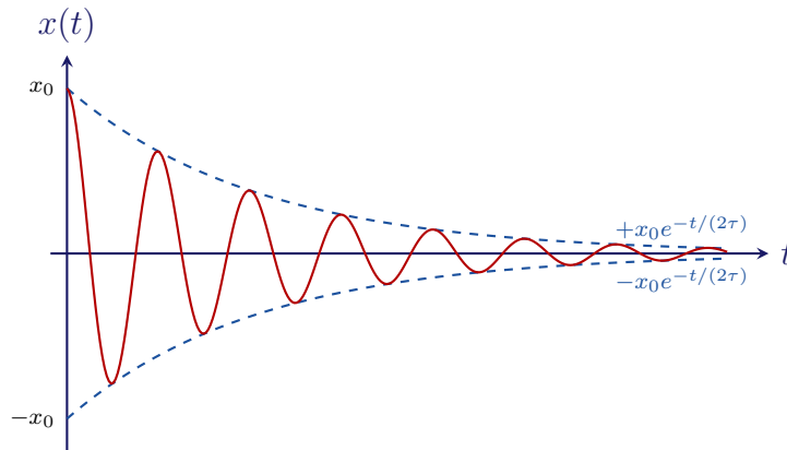
Figura 7.39: Andamento temporale di un'oscillazione smorzata sub-critica. L'ampiezza decade esponenzialmente con costante di tempo 2\tau .
