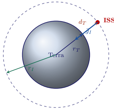
Figura 10.5: Geometria orbitale della Stazione Spaziale Internazionale. Alla quota d_T = 450 km il campo gravitazionale terrestre vale ancora circa l'86% del valore al suolo.
