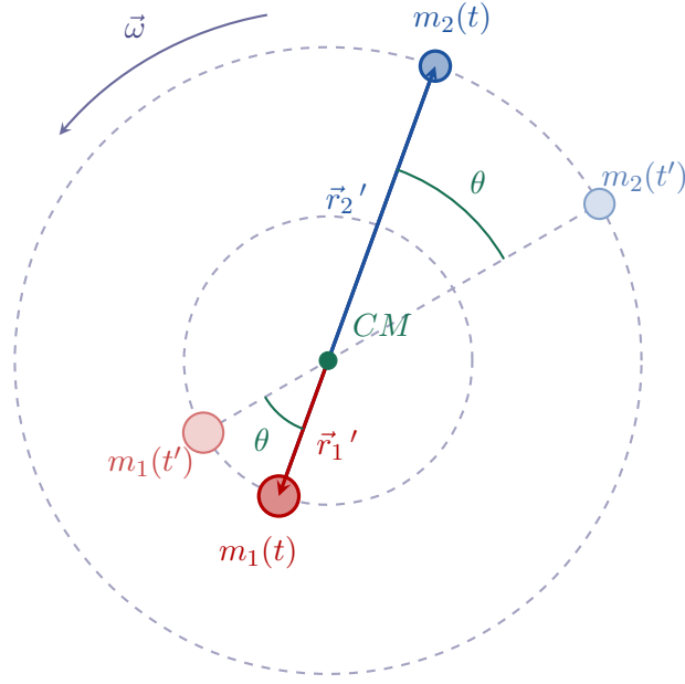
Figura 5.6: Orbite circolari in un sistema isolato a due corpi, ritratte in due istanti successivi t e t' . I due corpi restano costantemente allineati con il centro di massa e su lati opposti rispetto a esso, e spazzano nello stesso tempo il medesimo angolo \theta : la velocità angolare è comune. Il corpo più pesante ( m_1 ) percorre l'orbita di raggio minore.
