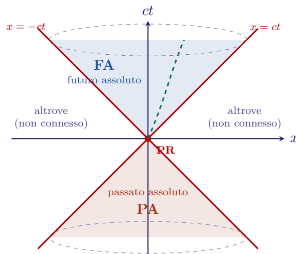
Figura 9.6: Il cono di luce di Minkowski. Solo gli eventi interni al cono sono causalmente connessi con l'evento nell'origine; la regione esterna ("altrove") raccoglie gli eventi per raggiungere i quali occorrerebbe una velocità superiore a c . La curva tratteggiata in verde è la linea di universo di un corpo che accelera restando sempre all'interno del cono.
