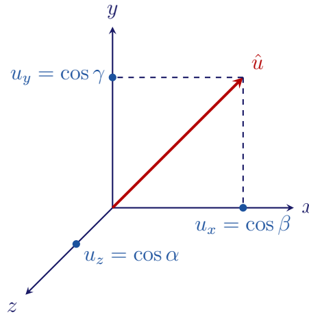
Figura 7.28: Rappresentazione spaziale del versore dell'asse di rotazione \hat{u} in termini dei suoi coseni direttori (u_x, u_y, u_z) in coordinate cartesiane.
