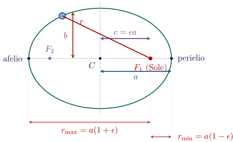
Figura 6.4: Geometria dell'orbita ellittica. Il Sole occupa il fuoco F_1 ; l'altro fuoco F_2 è vuoto. La distanza minima r_{\min} si raggiunge al perielio, quella massima r_{\max} all'afelio, e il semiasse maggiore a ne è la semisomma.
