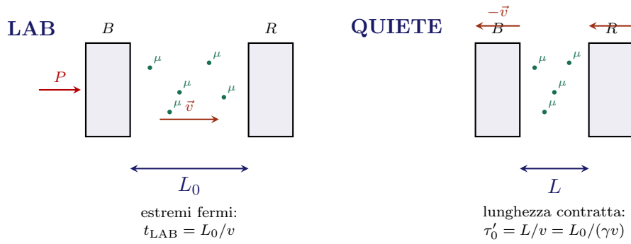
Figura 9.5: L'esperimento del muone letto nei due sistemi di riferimento. I protoni P colpiscono il bersaglio B producendo muoni, che percorrono la distanza fino al rivelatore R . Nel LAB la distanza è propria ( L_0 ) e il tempo dilatato; nel sistema di quiete del muone la distanza è contratta e il tempo è proprio.
