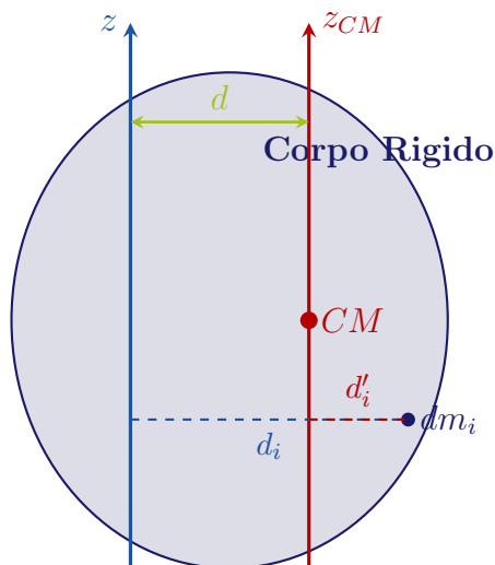
Figura 7.15: Geometria del Teorema di Huygens-Steiner: il momento d'inerzia rispetto a un asse arbitrario z è pari al momento d'inerzia rispetto all'asse parallelo passante per il centro di massa ( z_{CM} ) più il termine di traslazione Md^2 , dove d è la distanza ortogonale tra i due assi.
