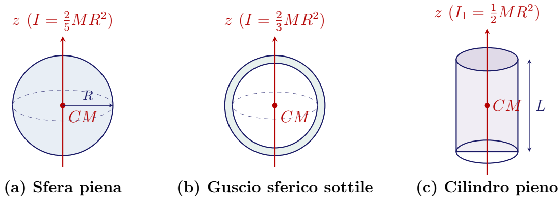
Figura 7.13: Momenti d'inerzia di corpi continui omogenei tridimensionali rispetto al loro asse principale d'inerzia di simmetria assiale.
