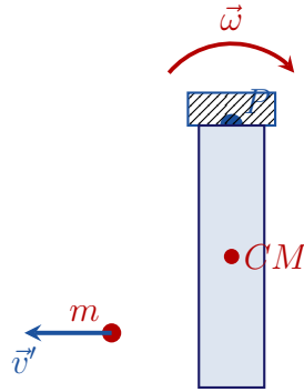
Figura 7.23: Nell'urto elastico con perno fisso P , il proiettile rimbalza con velocità \vec{v}' e la sbarretta entra in rotazione con velocità angolare \omega , senza alcuna dissipazione di energia cinetica.
