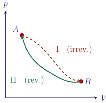
Figura 8.33: Ciclo impiegato per ricavare la disuguaglianza di Clausius in forma aperta: il sistema va da A a B lungo la trasformazione irreversibile I e ritorna da B ad A lungo la trasformazione reversibile II. Applicando \oint \delta Q/T < 0 al ciclo complessivo si ottiene \Delta S \geq \int_A^B \delta Q/T .
