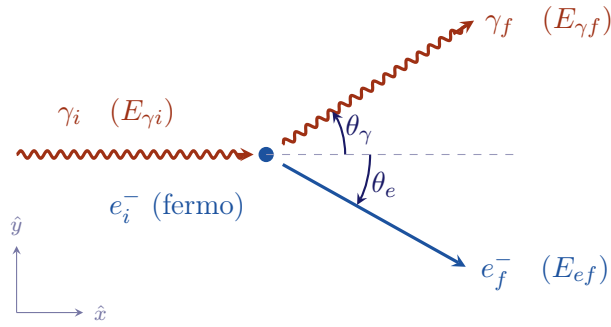
Figura 9.7: Cinematica dell'effetto Compton nel sistema del laboratorio: il fotone incidente \gamma_i viene diffuso di un angolo \theta_\gamma , mentre l'elettrone inizialmente fermo rincula di un angolo \theta_e .
