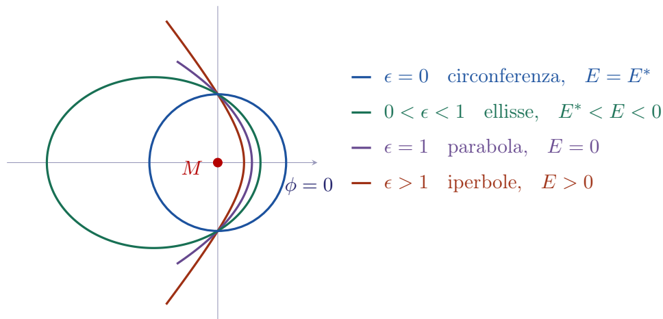
Figura 6.3: Le quattro famiglie di traiettorie in campo kepleriano, tutte con lo stesso semilato retto p e un fuoco comune nel centro di forza M . Al crescere dell'eccentricità — e quindi dell'energia — l'orbita passa da chiusa ad aperta.
