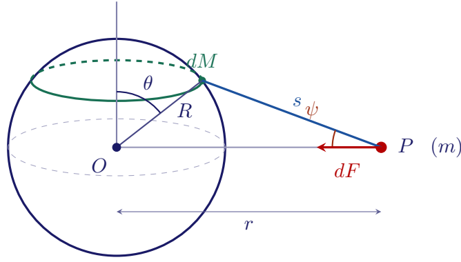
Figura 6.5: Geometria per il teorema dei gusci. Il guscio è suddiviso in anelli infinitesimi individuati dall'angolo \theta ; tutti i punti dell'anello distano s dal punto P , e le componenti trasversali delle forze si elidono per simmetria, lasciando la sola componente assiale dF \propto \cos \psi .
