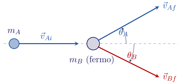
Figura 4.5: Scattering elastico in due dimensioni nel sistema del laboratorio, con il bersaglio m_B inizialmente fermo. Misurato uno dei due angoli di deflessione, le leggi di conservazione determinano univocamente l'altro angolo e i moduli delle due velocità finali.
