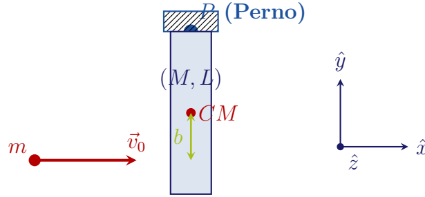
Figura 7.21: Urto tra un proiettile e una sbarretta vincolata a un perno fisso P in un estremo. Poiché il perno esercita una forza impulsiva esterna, la quantità di moto totale non si conserva, mentre si conserva il momento angolare rispetto al polo fisso P .
