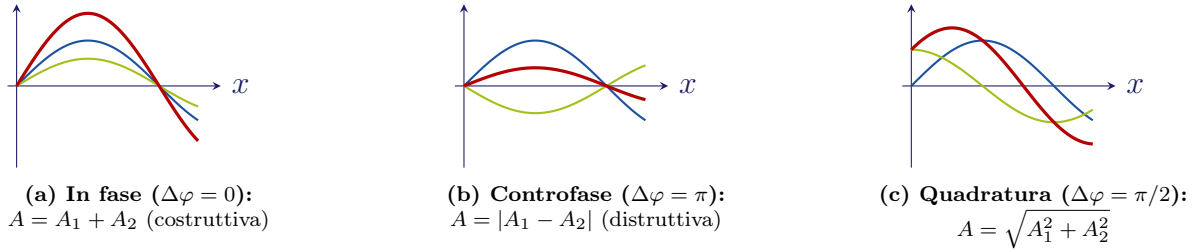
Figura 7.36: Interferenza tra due moti armonici paralleli isocroni di ampiezza differente ( A_1 \neq A_2 ). La curva risultante è riportata in rosso.
