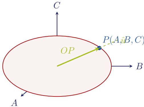
Figura 7.30: Rappresentazione geometrica dell'ellissoide d'inerzia: la distanza OP dall'origine al generico punto sulla superficie lungo la direzione \hat{u} è pari al reciproco della radice quadrata del momento d'inerzia lungo quell'asse ( OP = 1/\sqrt{I_u} ).
