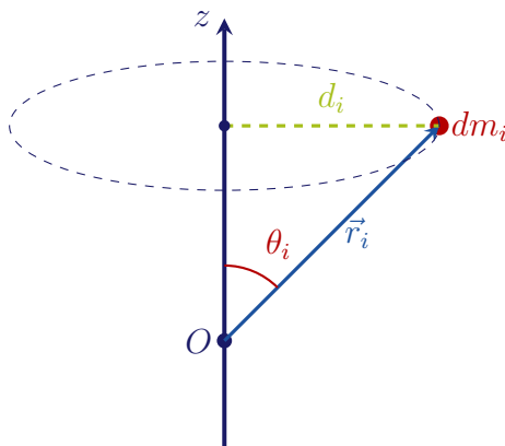
Figura 7.16: Rotazione di un elemento di massa dm_i attorno ad un asse fisso z : la distanza dall'asse di rotazione è data dalla proiezione ortogonale d_i = r_i \sin \theta_i .
