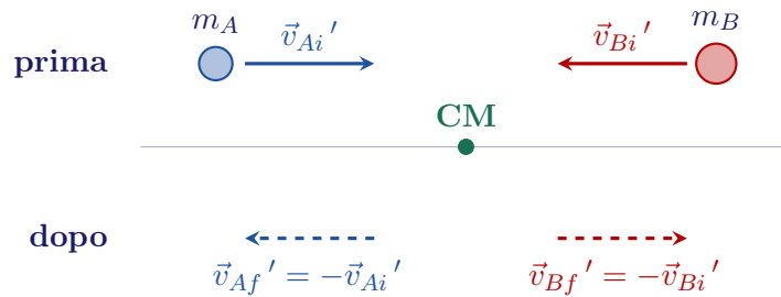
Figura 4.6: Urto elastico unidimensionale nel sistema del centro di massa. I due corpi si avvicinano con quantità di moto uguali e opposte e si rallontanano con le stesse quantità di moto invertite: l'urto si riduce a un cambio di segno.
