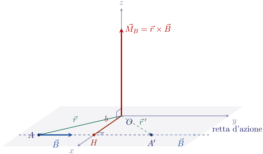
Figura 5.1: Momento del vettore \vec{B} rispetto al polo O . I punti A e A' sono due scelte arbitrarie del punto di applicazione lungo la stessa retta d'azione: il momento \vec{M}_B , ortogonale al piano individuato da \vec{r} e \vec{B} , è il medesimo in entrambi i casi e il suo modulo vale |\vec{B}| b , dove b è il braccio.
