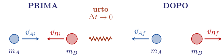
Figura 4.1: Struttura logica di un urto. L'interazione vera e propria, confinata in un intervallo \Delta t \rightarrow 0 , viene trattata come una scatola nera: si confrontano soltanto lo stato iniziale e lo stato finale. La quantità di moto totale si conserva in ogni caso, \vec{P}_f = \vec{P}_i ; l'energia cinetica soltanto se l'urto è elastico.
