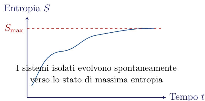
Figura 8.34: Andamento nel tempo dell'entropia di un sistema isolato.
