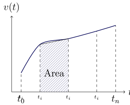
Figura 1.5: Interpretazione geometrica dell'integrale come area sottesa al grafico.
