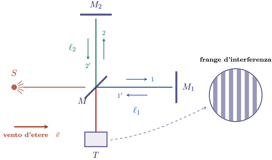
Figura 9.2: Schema dell'interferometro di Michelson. La sorgente S invia il raggio sullo specchio semiriflettente M , che lo divide nei due raggi 1 e 2 diretti agli specchi M_1 e M_2 lungo i bracci \ell_1 e \ell_2 ; i raggi riflessi 1' e 2' si ricombinano nel telescopio T , dove producono le frange d'interferenza.
