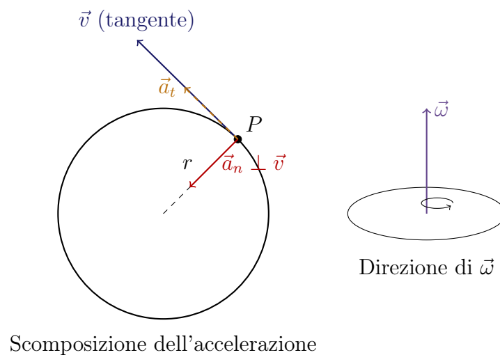
Figura 1.8: Cinematica del moto circolare.
