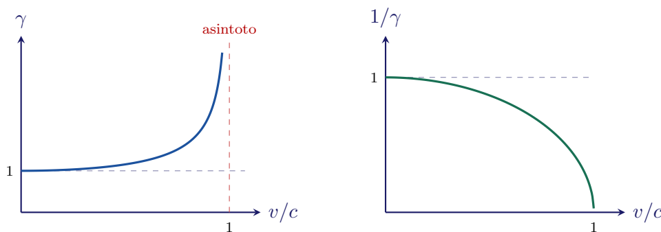
Figura 9.4: Andamento del fattore di Lorentz \gamma e del suo reciproco 1/\gamma in funzione di \beta = v/c . Il fattore \gamma diverge per v \rightarrow c , mentre 1/\gamma (il fattore di contrazione) si annulla nello stesso limite.
