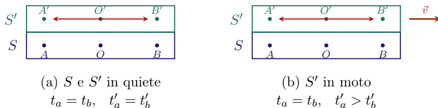
Figura 9.3: La relatività della simultaneità. Due eventi simultanei nel sistema S non lo sono più nel sistema S' in moto: l'osservatore O' va incontro al segnale proveniente da B e si allontana da quello proveniente da A .
