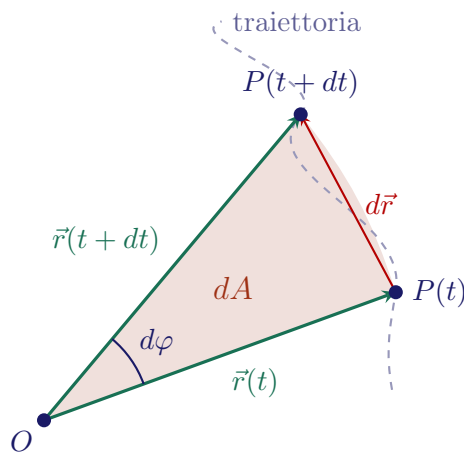
Figura 5.4: Interpretazione geometrica della costanza del momento angolare: nell'intervallo dt il raggio vettore spazza l'area infinitesima dA , assimilabile a un settore circolare di ampiezza d\varphi .
