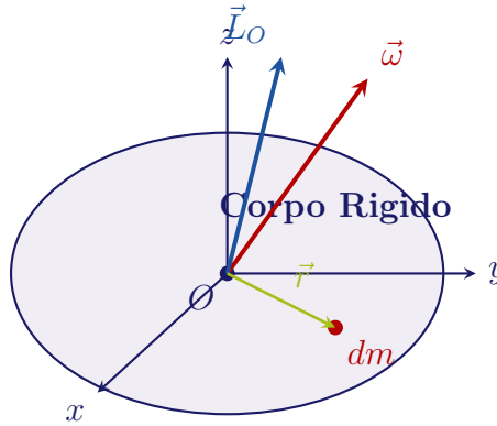
Figura 7.27: In un corpo rigido generale in rotazione attorno ad un asse arbitrario passante per O , il momento angolare \vec{L}_O non è in generale parallelo alla velocità angolare \vec{\omega} . La relazione lineare tra i due vettori è descritta dal tensore d'inerzia \mathbf{I} .
