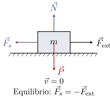
Figura 2.11: Attrito Statico: si oppone alla forza motrice finché il corpo è fermo.
