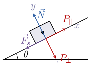
Figura 2.13: Equilibrio limite su piano inclinato.
