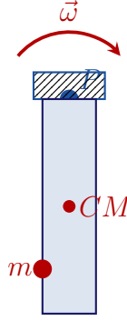
Figura 7.22: Nell'urto anelastico con sbarretta vincolata al perno P , il proiettile rimane conficcato nella sbarretta, ponendo l'intero sistema in pura rotazione attorno a P con velocità angolare \omega .
