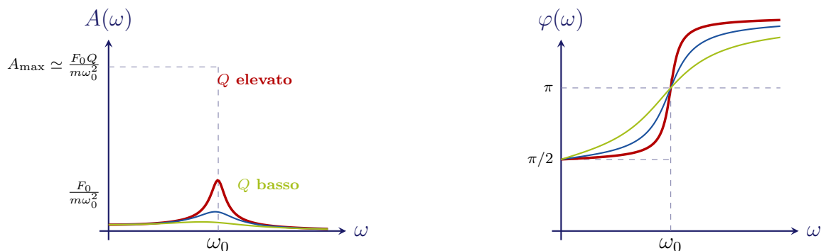
(a) Curva di risonanza dell'ampiezza A(\omega)
