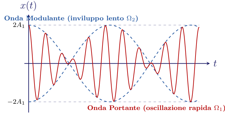
Figura 7.37: Rappresentazione del fenomeno dei battimenti: un'onda rapida la cui ampiezza varia lentamente nel tempo.
