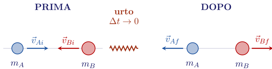
Figura 4.1: Struttura logica di un urto. L'interazione vera e propria, confinata in un intervallo \Delta t \rightarrow 0 , viene trattata come una scatola nera: si confrontano soltanto lo stato iniziale e lo stato finale. La quantità di moto totale si conserva in ogni caso, \vec{P}_f = \vec{P}_i ; l'energia cinetica soltanto se l'urto è elastico.
