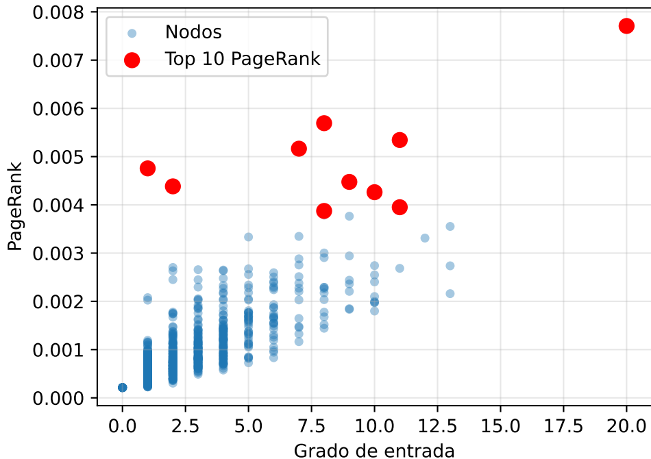
PageRank vs. grado de entrada ( r=0.797 )
