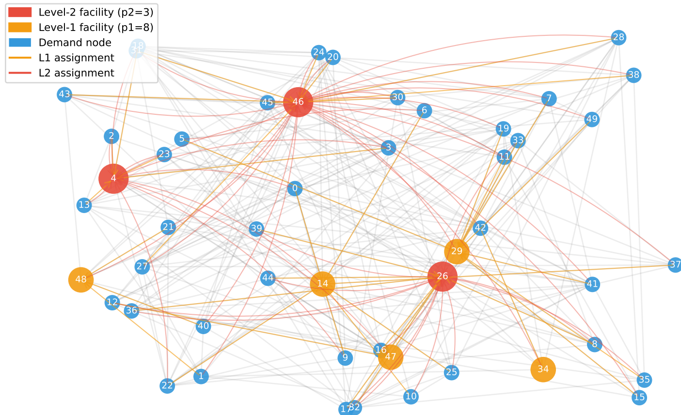
SA Solution - Random Graph (n=50) cost=176.21
