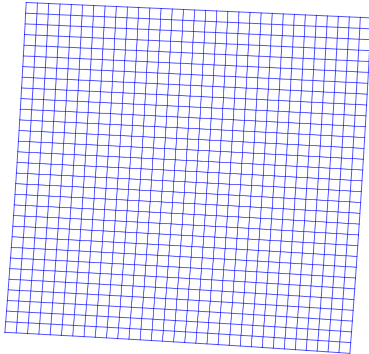
Dominio Fisico Mappato \phi(\Omega_I)
