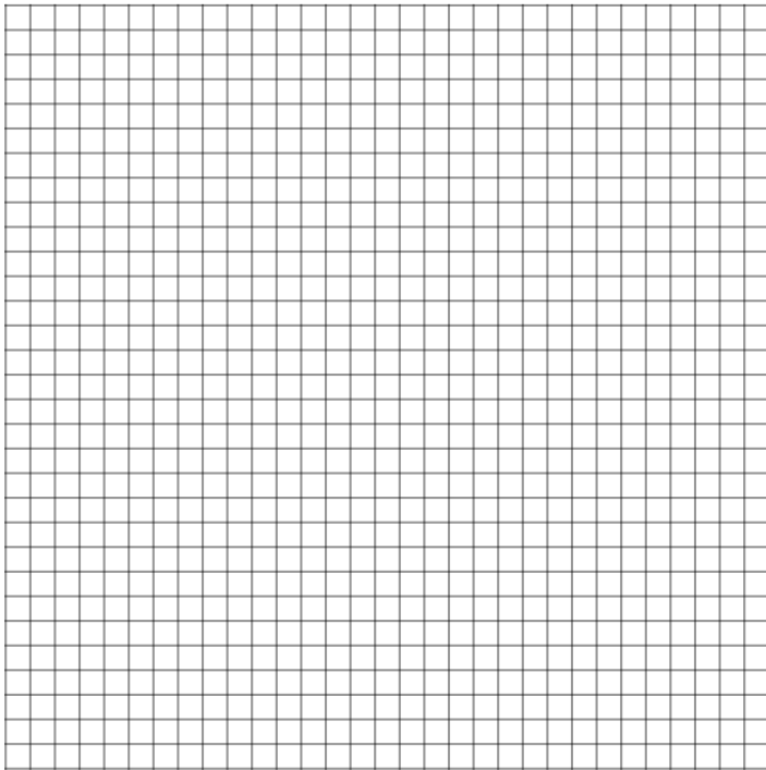
Dominio Latente \Omega_I (Canónico)
