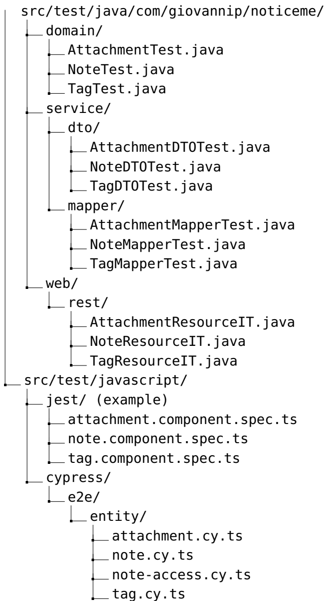
Figura 3: Estratto dell'albero dei test generati automaticamente
