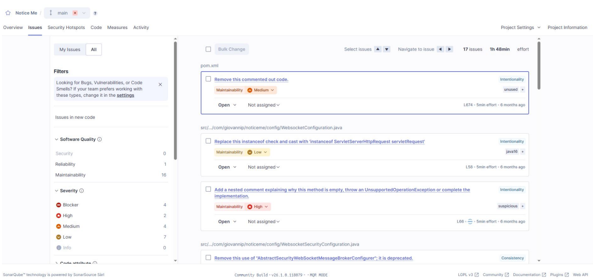
Figura 11: Sezione Issues di SonarQube con i problemi individuati dall'analisi statica del codice.
