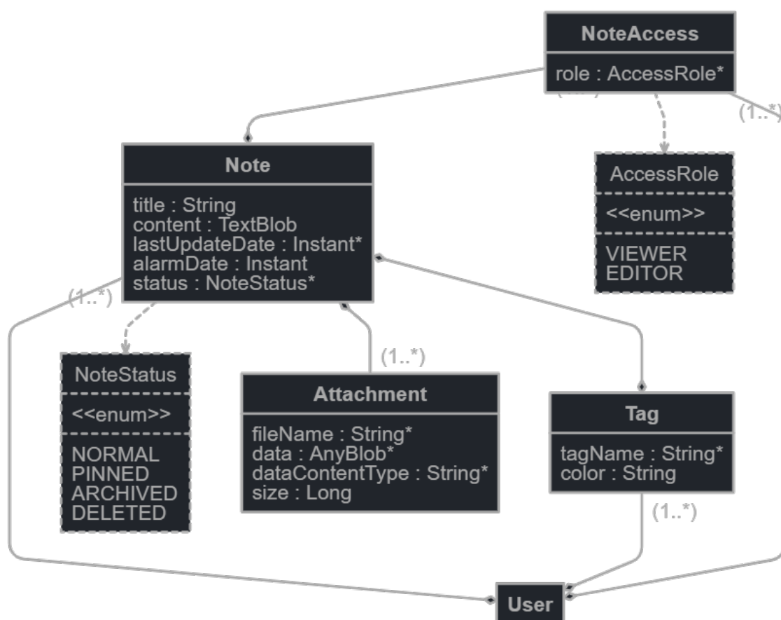
Figura 2: Schema concettuale del dominio e relazione multi-a-molti tra note e tag.
