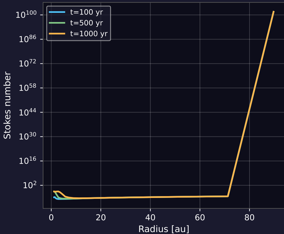
Stokes number ( \alpha = 10^{-3} , 0.05 M_{\odot} disc)
