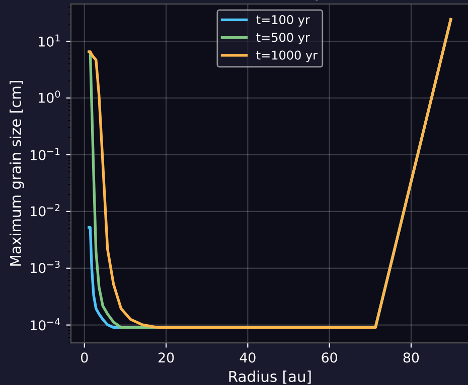
Grain size evolution ( v_{\text{frag}}=10 \text{ m s}^{-1} )
