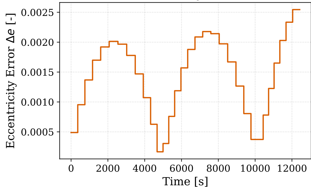
Eccentricity Error
