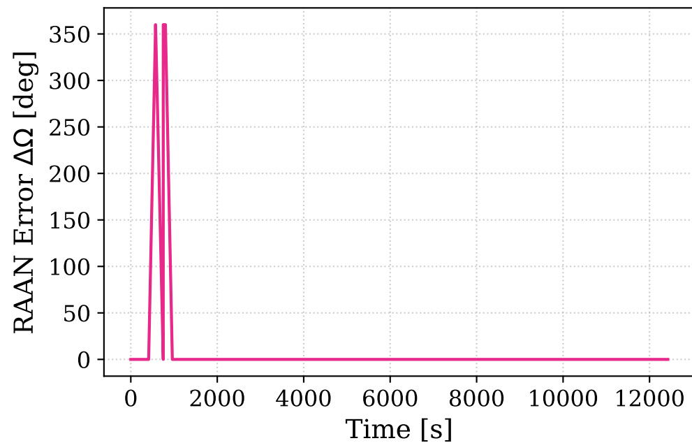
RAAN Error
