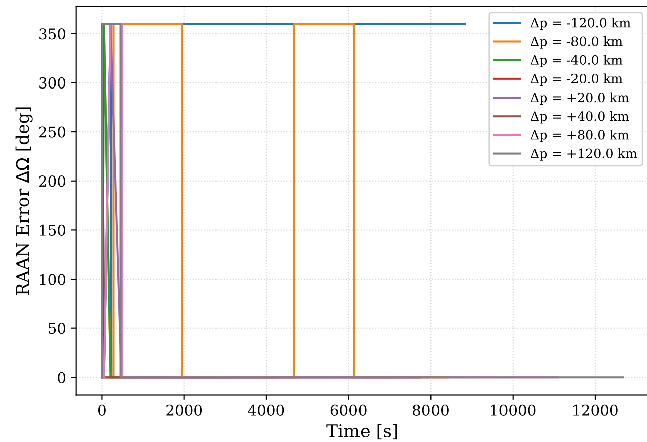
(d) RAAN Error \Delta \Omega
