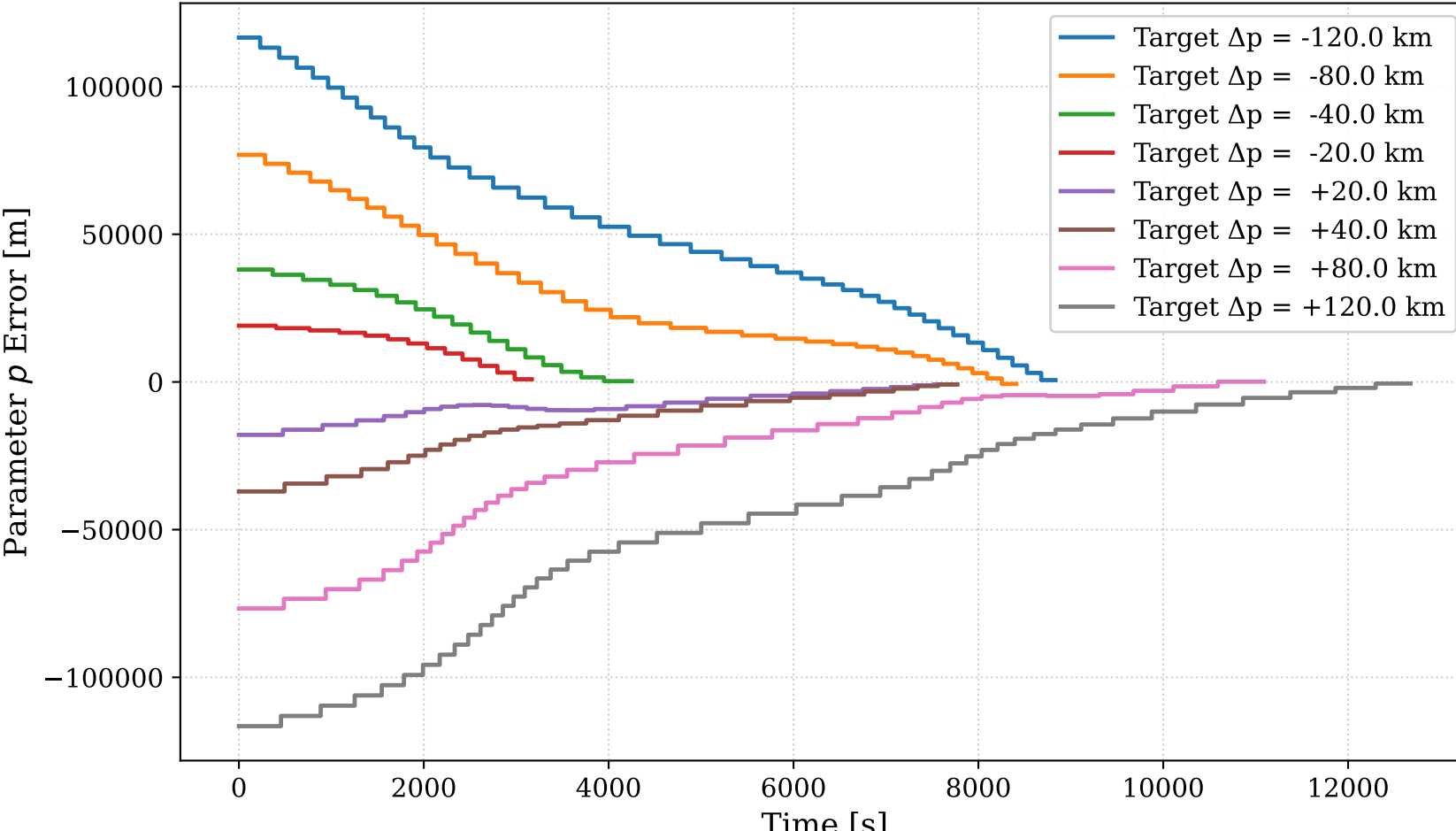
Zero-Shot Parameter p Error Trajectories Across Test Orbits
