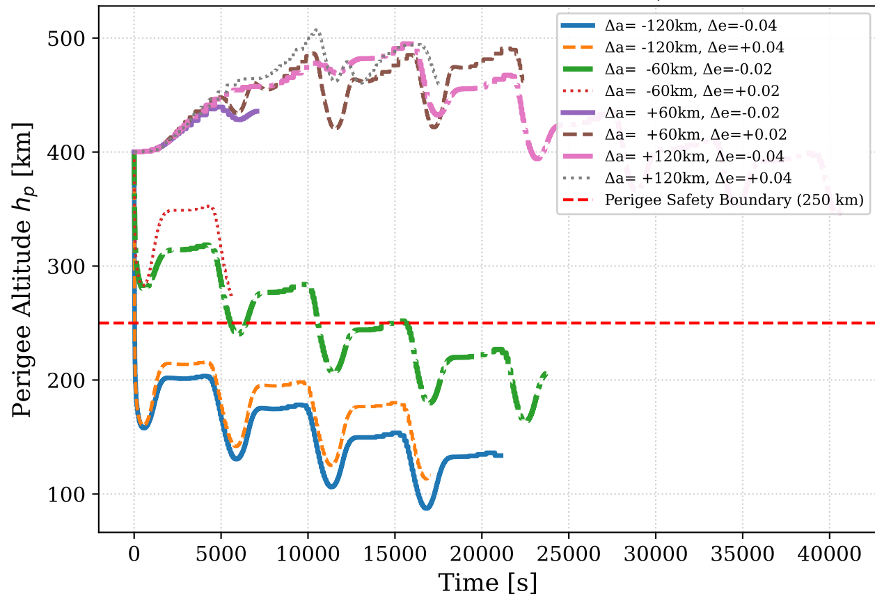
Perigee Altitude Evolution ( h_p )
