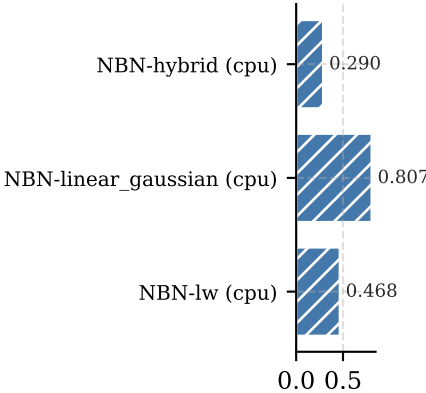
(d) Hybrid — W_1 vs filtered SCM samples
