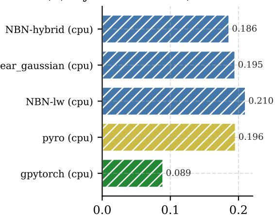
(d) Hybrid — MAE (mean vs MC ref)
