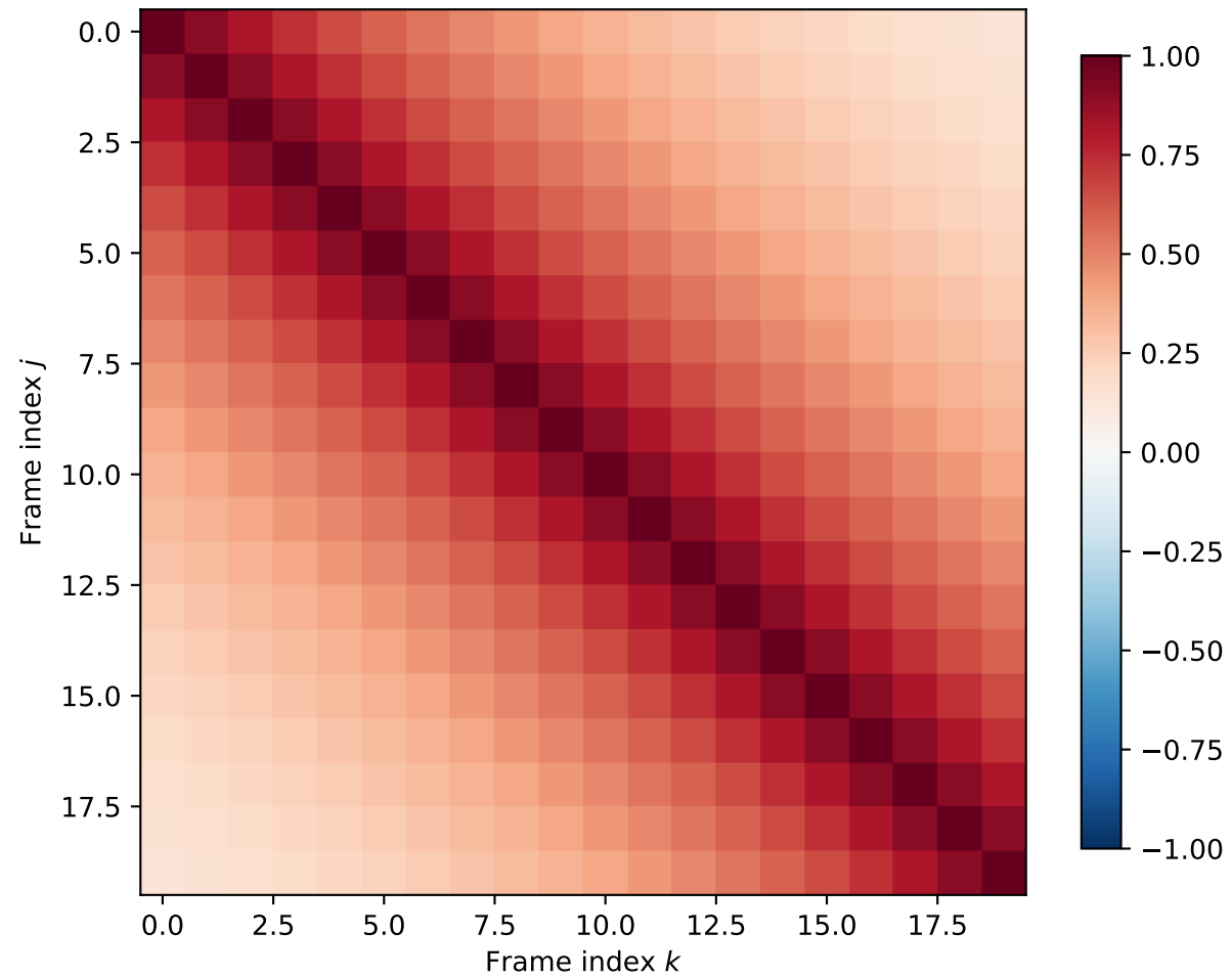
\Sigma_0 (Covariance — Dense)
