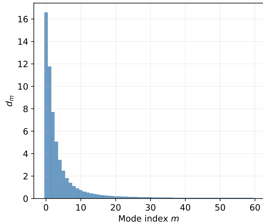
Eigenvalues of \Sigma_0
