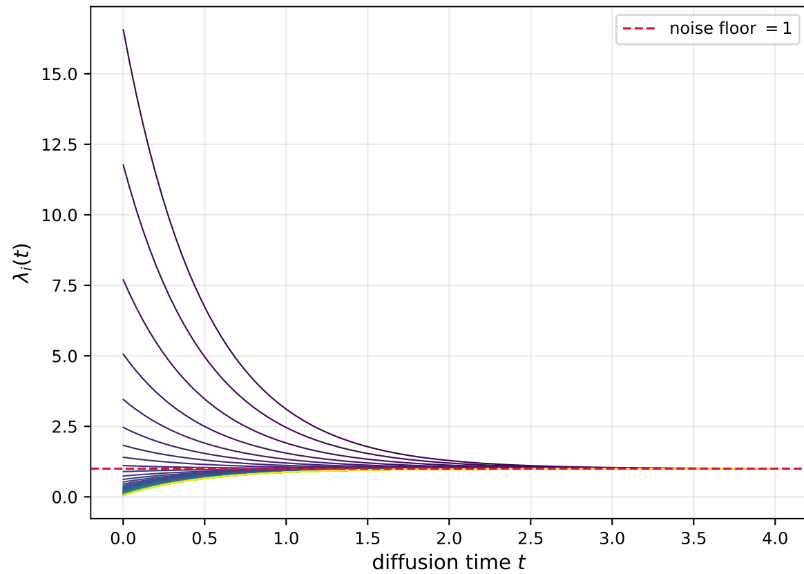
Eigenvalues of \Sigma_t
