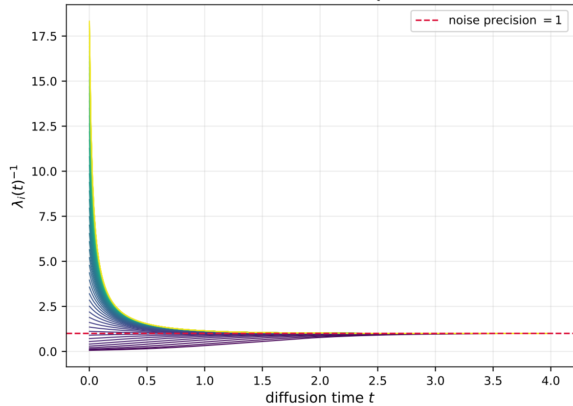
Eigenvalues of \Sigma_t^{-1}
