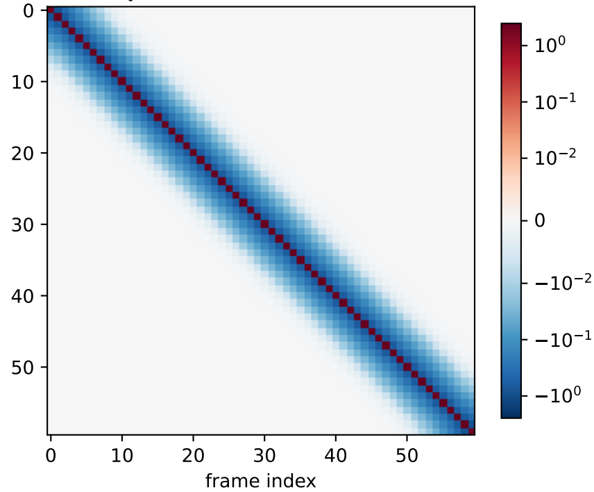
\Sigma_t^{-1} , symlog scale, t = 0.15
