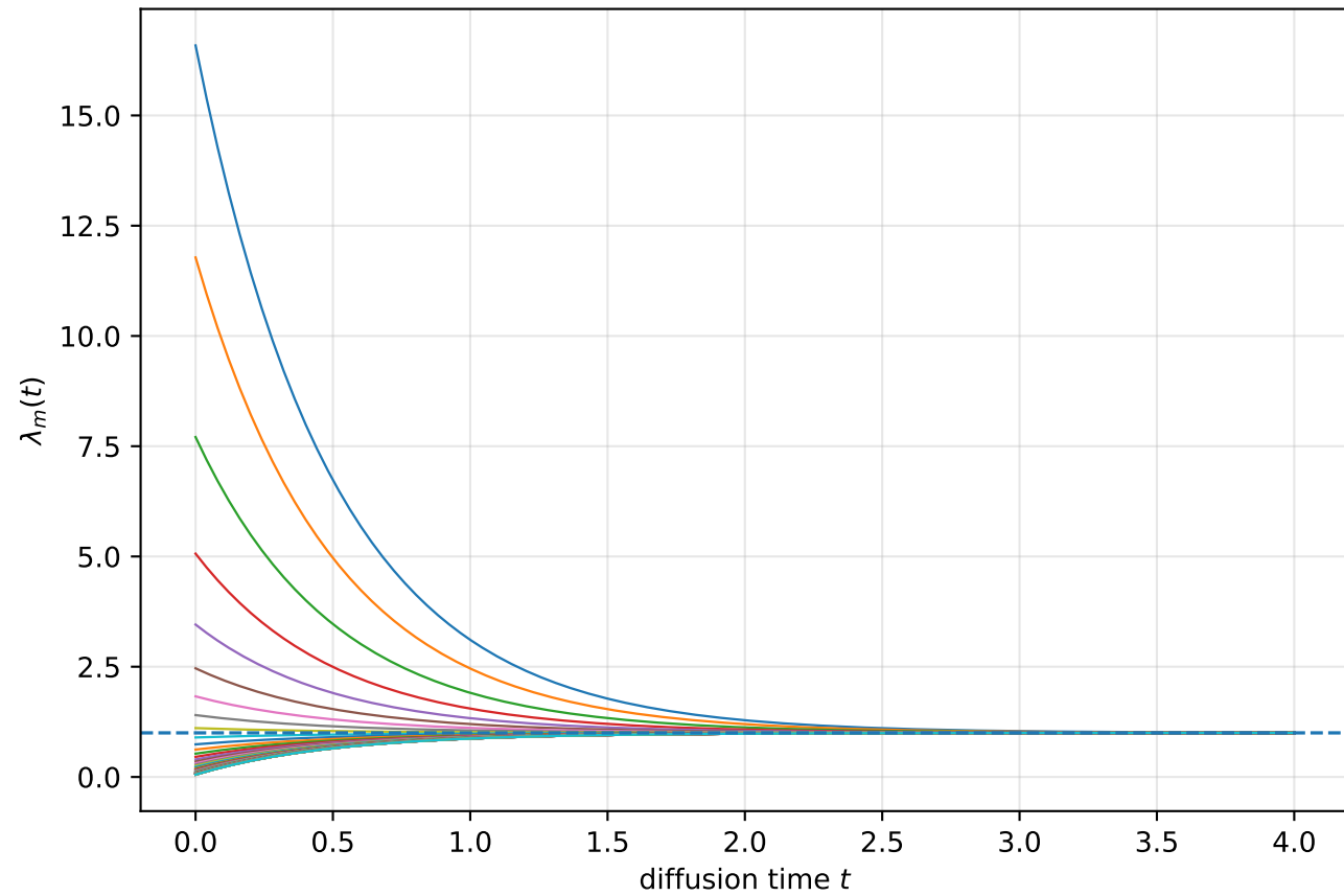
eigenvalues of \Sigma_t
