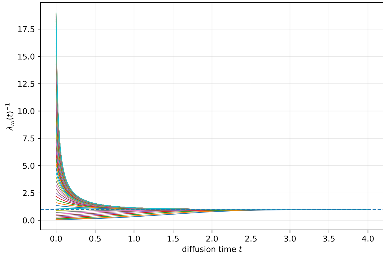
eigenvalues of \Sigma_t^{-1}
