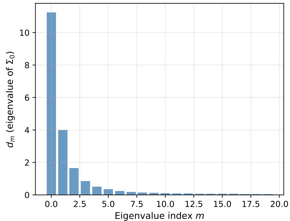
Eigenvalues of \Sigma_0
