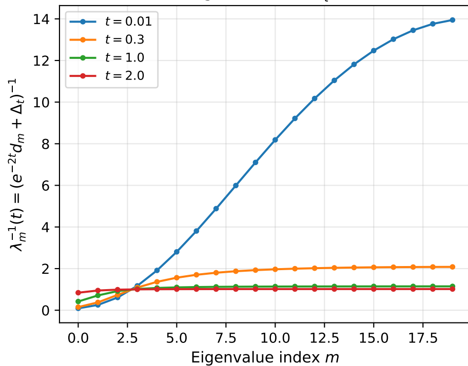
Eigenvalues of \Sigma_t^{-1}
