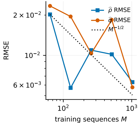
parameter recovery
