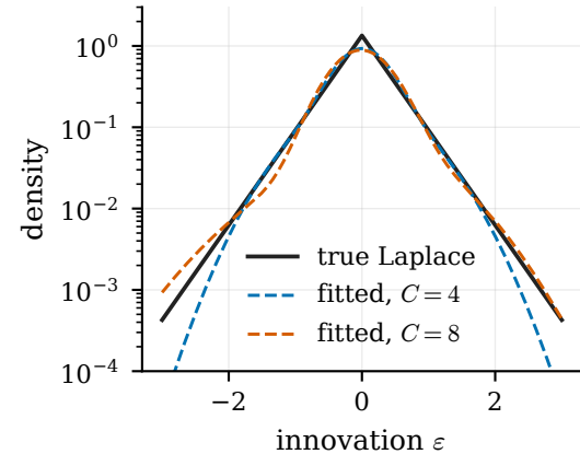
128 EM updates
