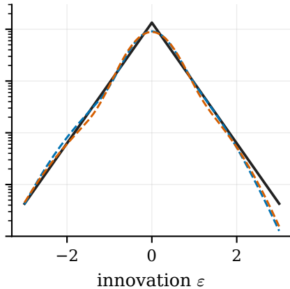
512 EM updates
