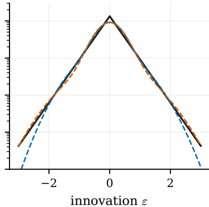
2048 EM updates
