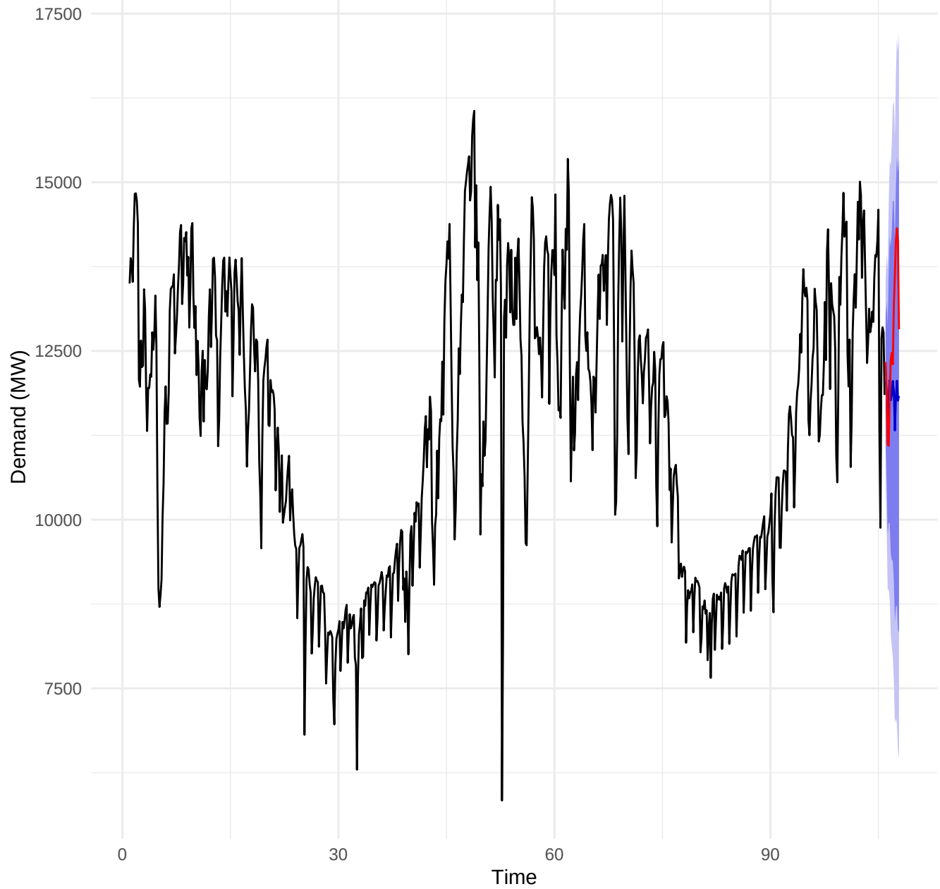
Holt-Winters Forecast vs Actual
