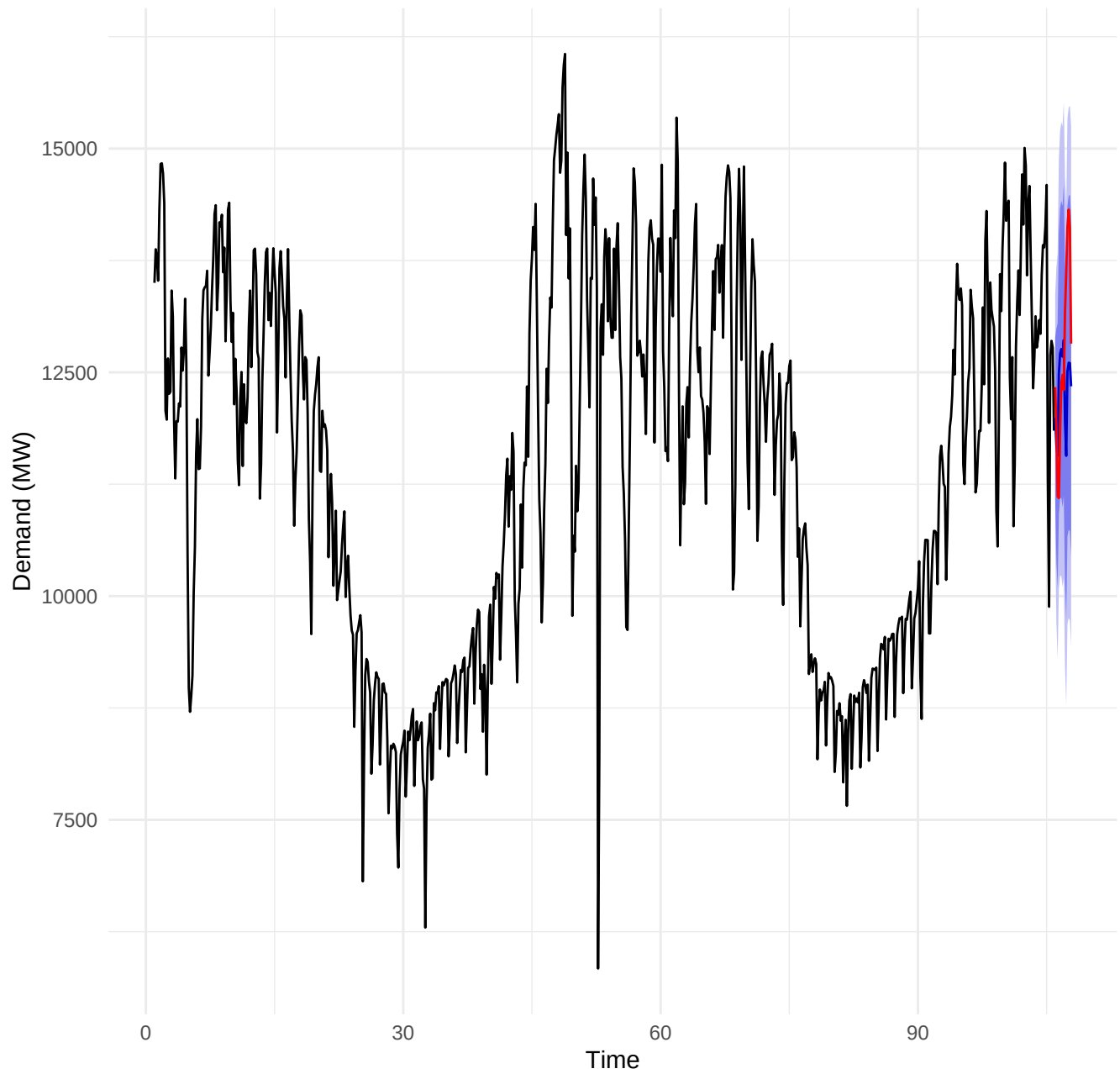
SARIMA Forecast vs Actual
