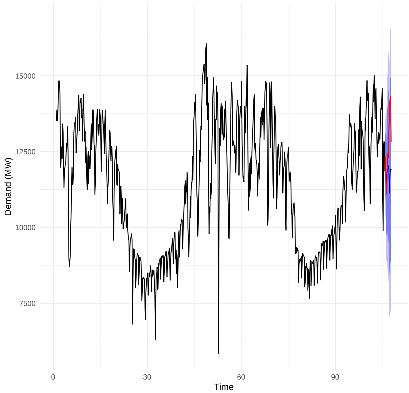
ETS Forecast vs Actual
