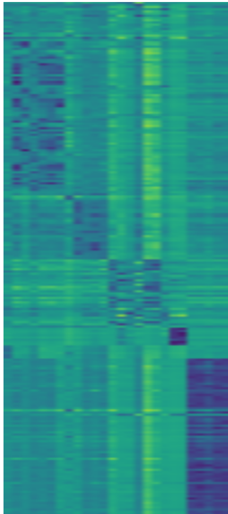
NObootstrap_sim50
