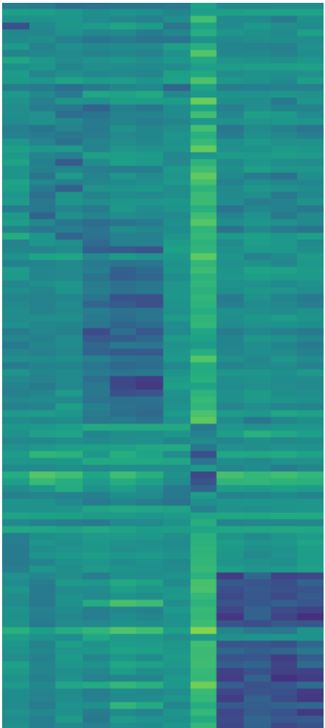
NObootstrap_sim40
