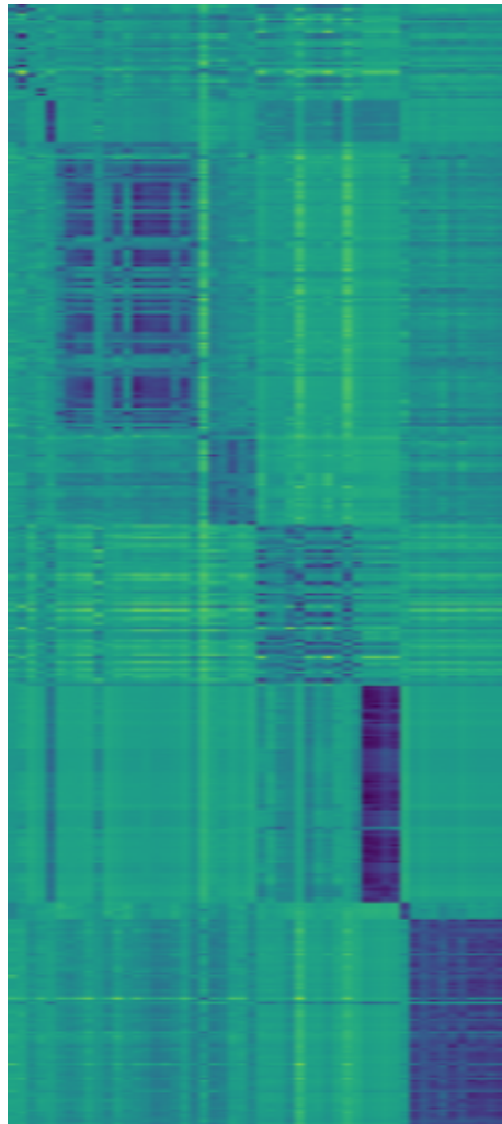
NObootstrap_sim70
