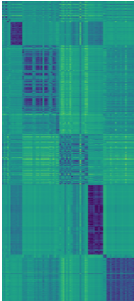
NObootstrap_sim80
