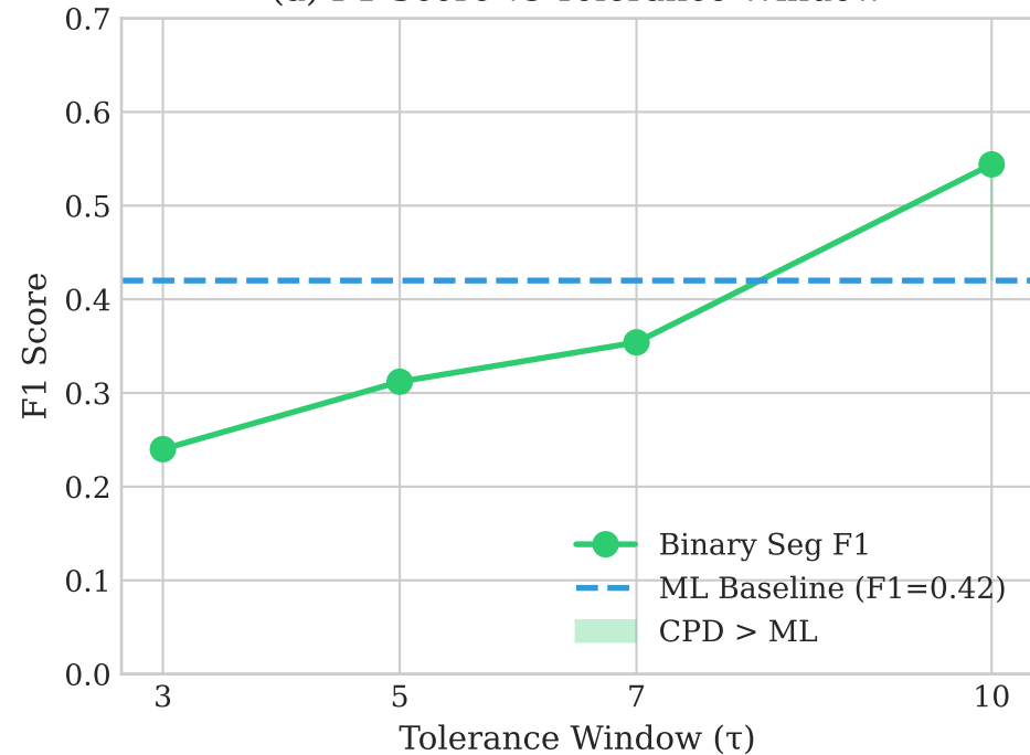
(a) F1 Score vs Tolerance Window
