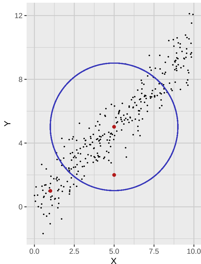
Figura 4.3: Dispersión con vector de media muestral y un círculo de distancia euclidiana constante al centro de los datos.
