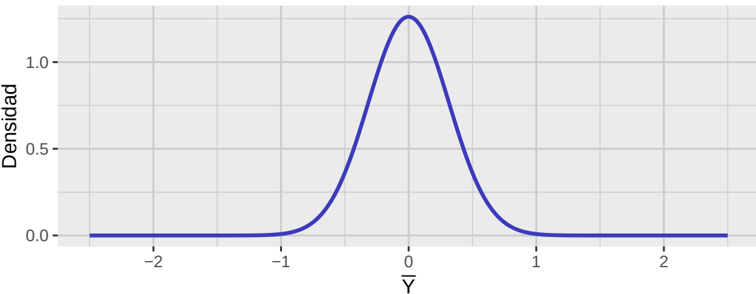
Densidad de \bar{Y}
