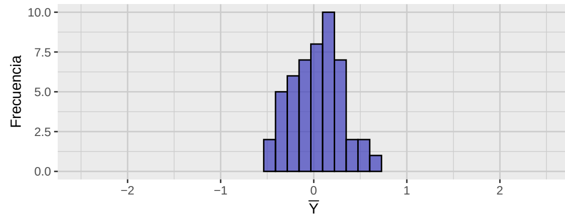
Muestra de tamaño 50 de \bar{Y}
