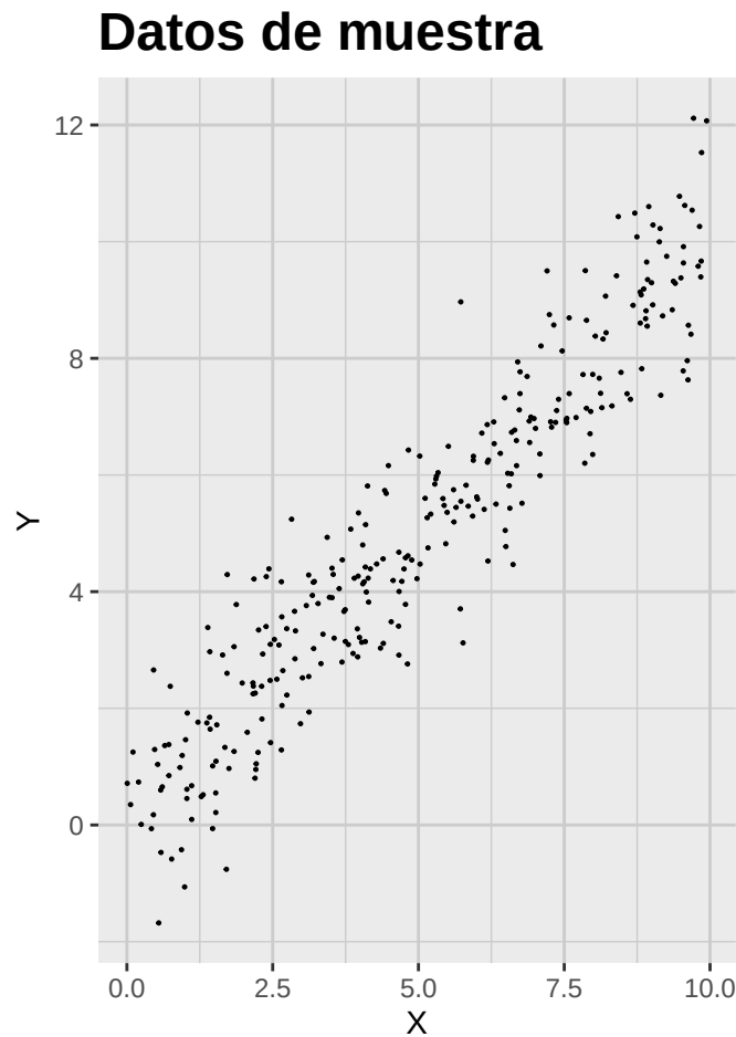
Figure 6.1: Datos de muestra con dos variables altamente correlacionadas.
