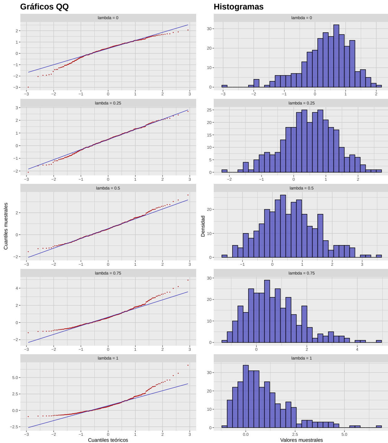
Figure 3.1: Comparación de distintas transformaciones de Box-Cox aplicadas a la muestra Gamma, con parámetro \lambda = 0, 0.25, 0.5, 0.75 y 1.
