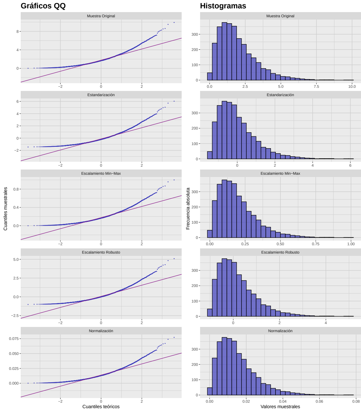
Figura 3.2: Comparación de distintos métodos de escalamiento aplicados a una muestra generada a partir de la distribución Gamma. Notemos que todos los gráficos QQ son versiones reescaladas del gráfico QQ original y, por tanto, tienen la misma forma. En particular, no es posible alterar la normalidad de una muestra al aplicar un método de escalamiento.
