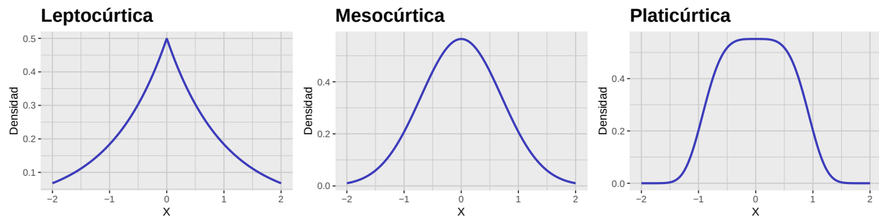
Figura 2.4: Gráfica comparativa de distribuciones leptocúrtica, mesocúrtica y platicúrtica. Notemos cómo la curtosis afecta la forma de la distribución, especialmente en las colas y el pico central.
