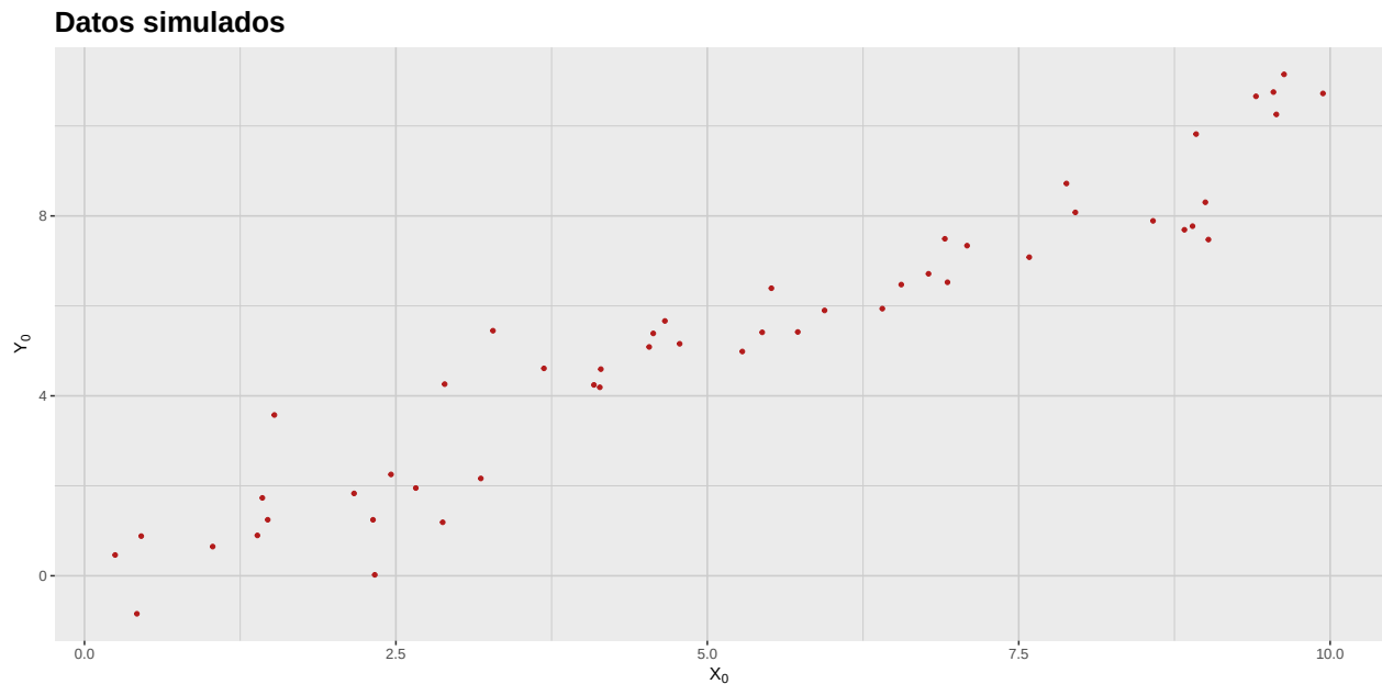
Figura 1.1: Diagrama de dispersión de los datos simulados.
