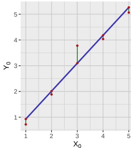
Figura 1.3: Ajuste por mínimos cuadrados para el conjunto de datos del ejemplo.
