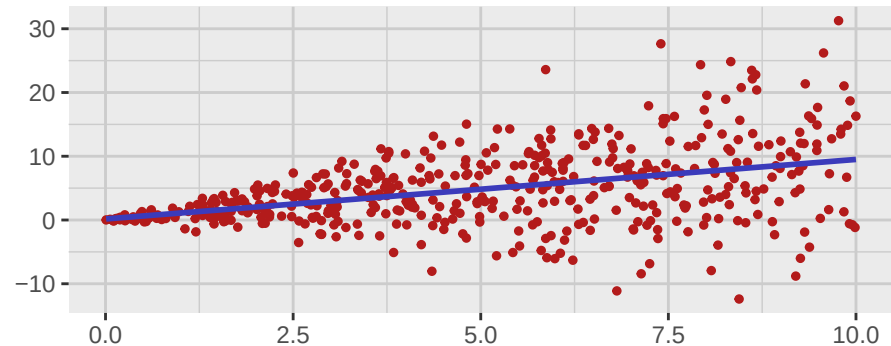
Datos con varianza creciente
