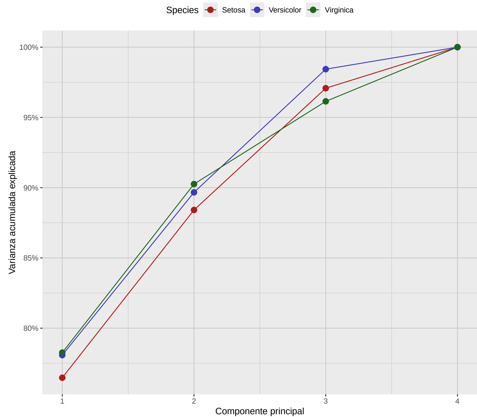
Varianza acumulada explicada por los componentes principales
