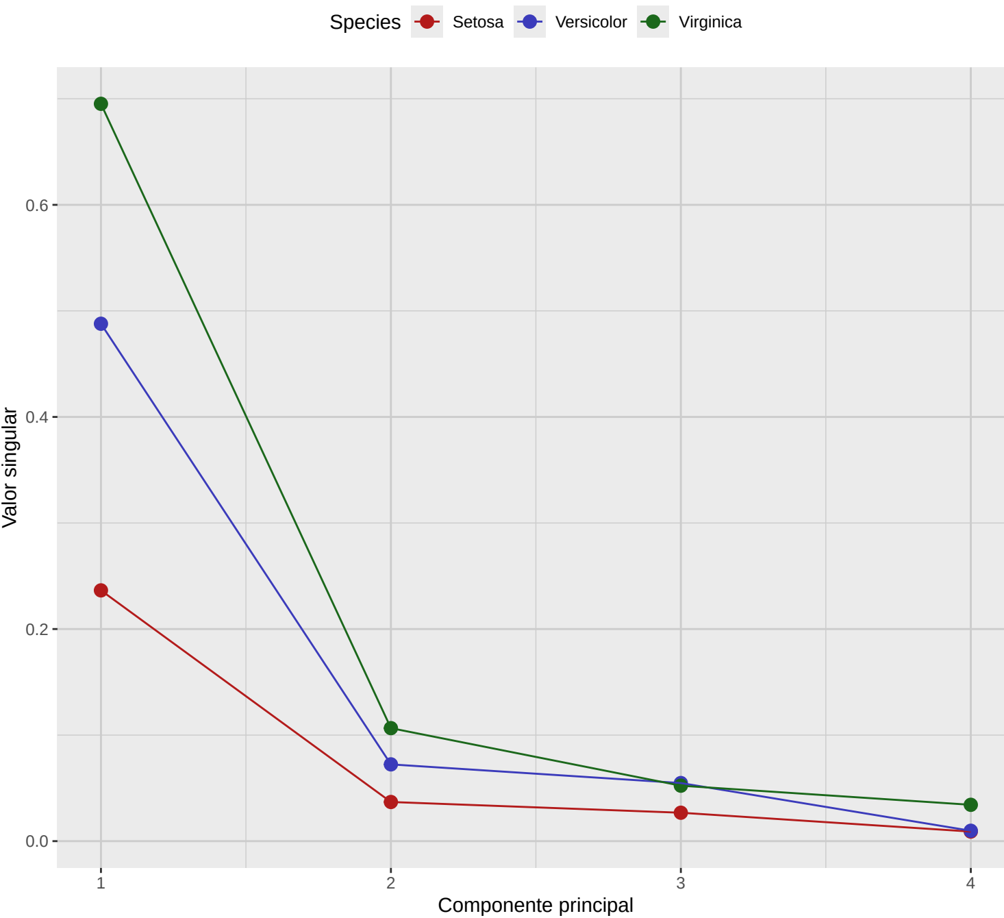
Gráfico scree del conjunto Iris
