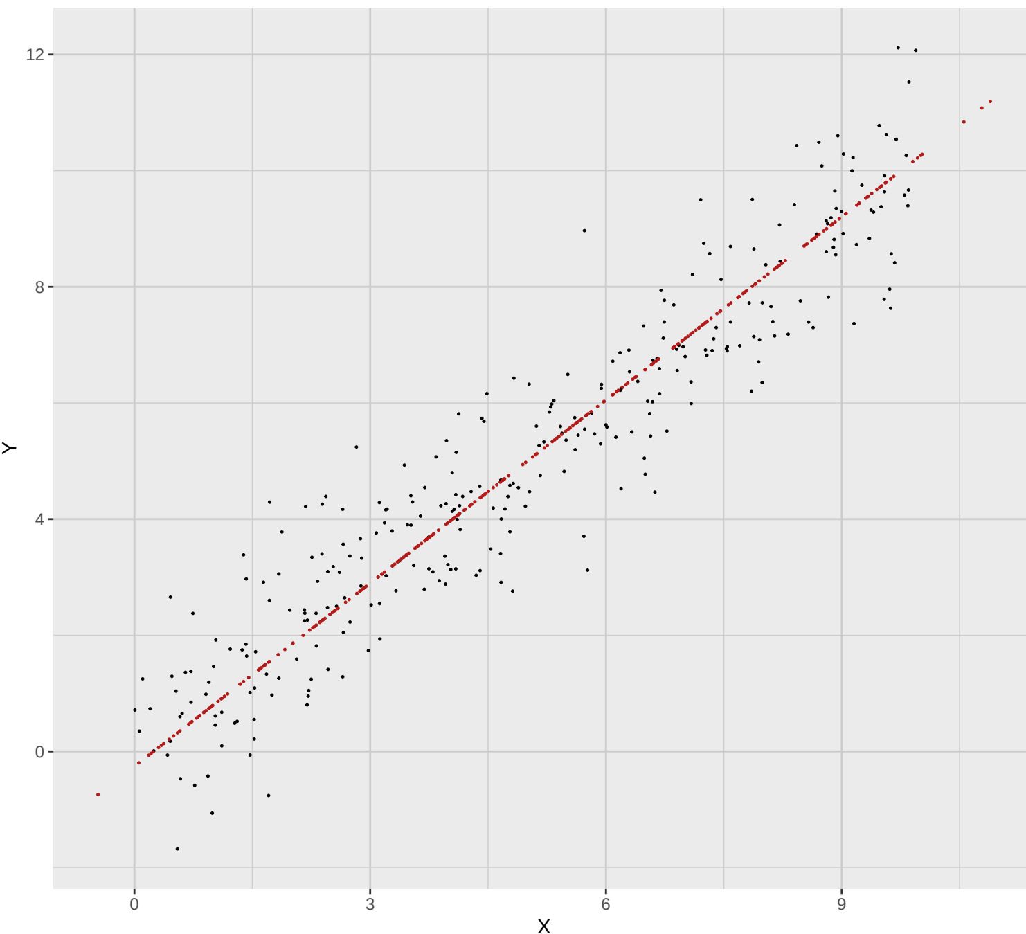
Proyección en el primer componente principal
