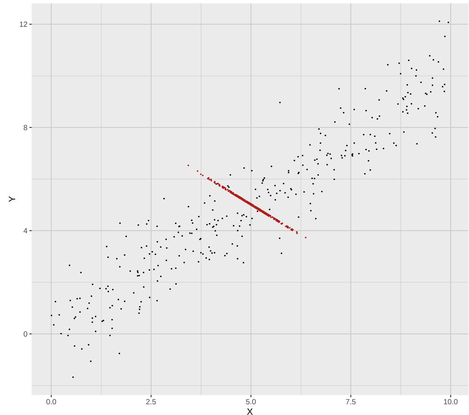
Proyección en el segundo componente principal
