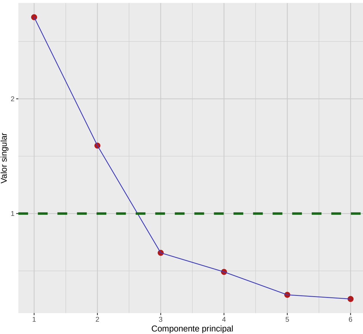
Gráfico scree
