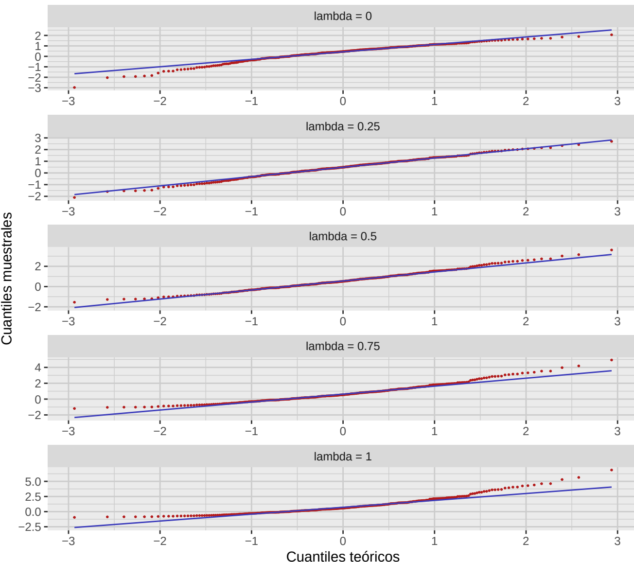
Gráficos QQ
