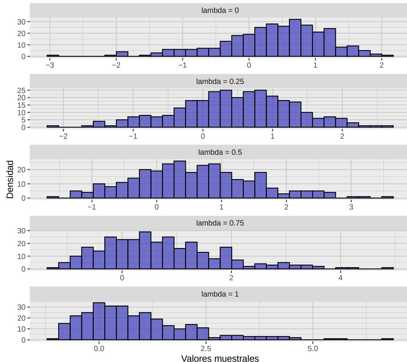
Histogramas
