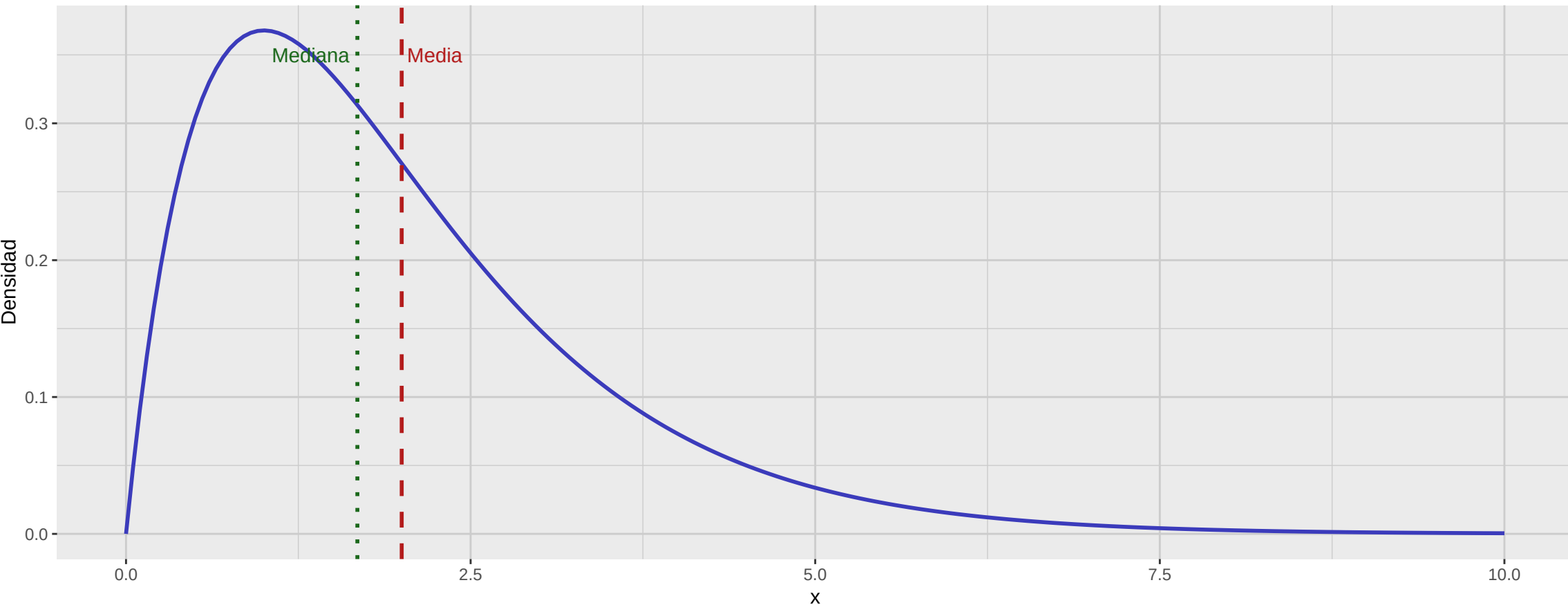
PDF de la distribución Gamma (shape = 2 , rate = 1 )
