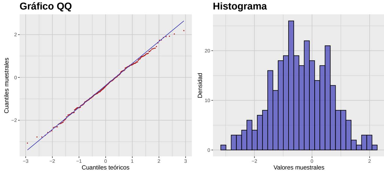
Figura 4.3: Gráfico QQ e histograma de la transformación Gamma óptima. Nótese el mejor ajuste a la normalidad en comparación con la muestra Gamma original.
