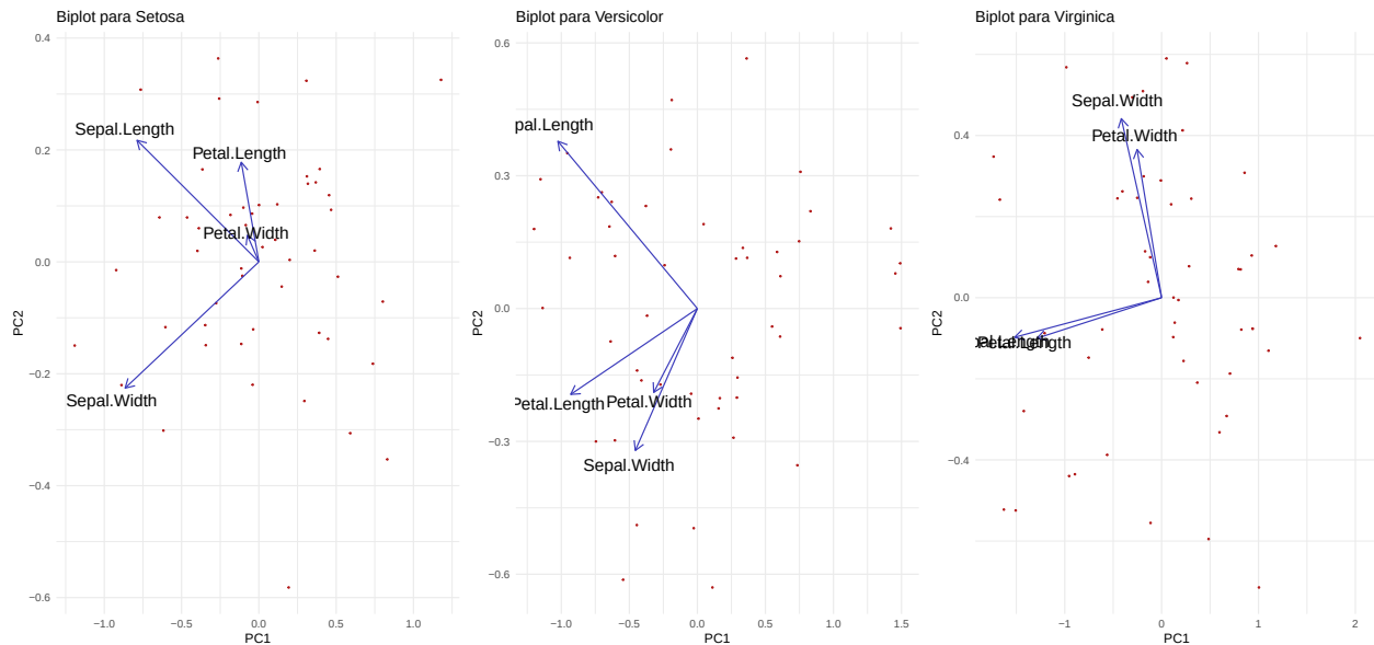
Figura 7.4: Cargas y puntuaciones para los dos primeros componentes principales del conjunto Iris por especie.
