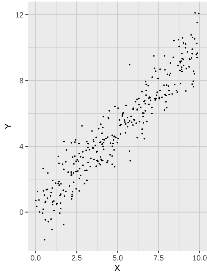
Figura 7.1: Datos de muestra con dos variables altamente correlacionadas.
