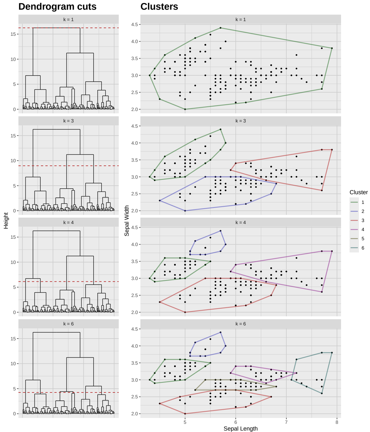
Figura 10.2: Agrupamiento jerárquico del conjunto de datos Iris considerando únicamente las variables 'Sepal.Length' y 'Sepal.Width'. Las líneas punteadas indican los puntos de corte para los números de clústeres dados ( k = 1, 3, 4, 6 ).
