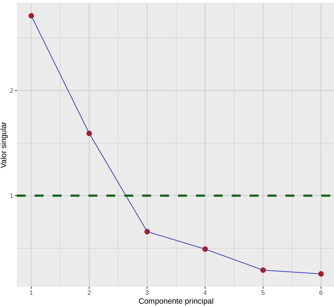
Gráfico scree
