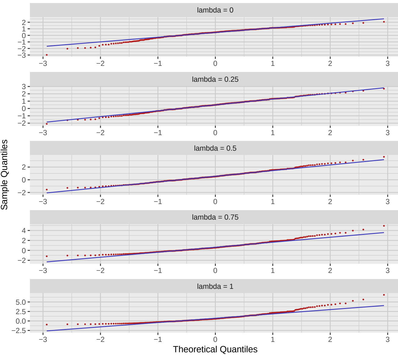
QQ Plots
