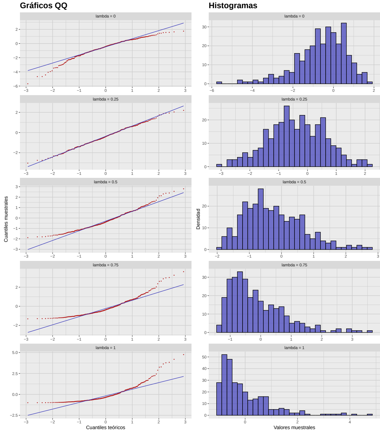
Figura 3.3: Comparación de distintas transformaciones de Box-Cox aplicadas a la muestra Gamma, con parámetro \lambda = 0, 0.25, 0.5, 0.75 y 1 .
