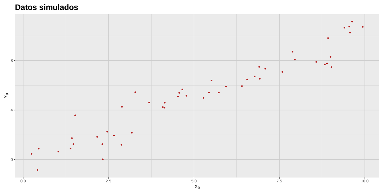
Figura 1.1: Diagrama de dispersión de los datos simulados.
